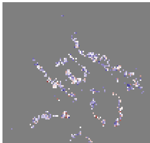
n_A _final
