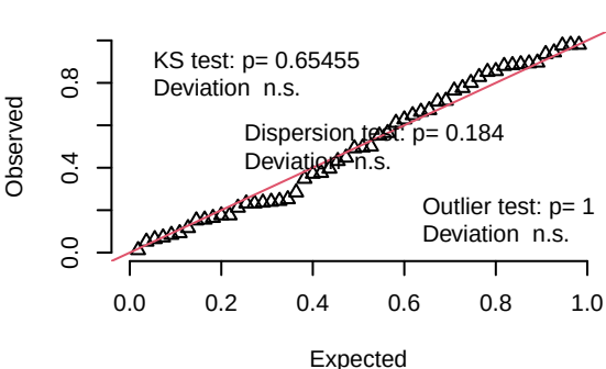
(F) P(n_S > 0)
