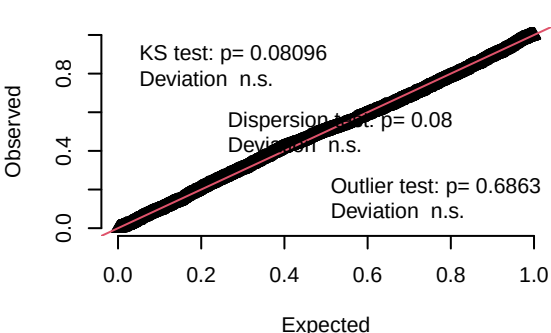
(D) P(n_R > 0)
