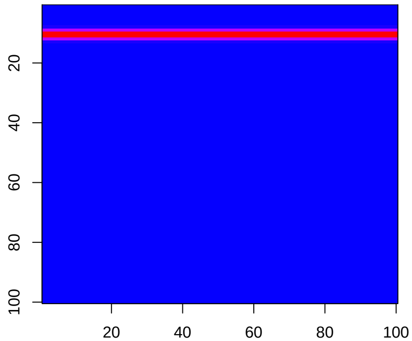
F subkernel
