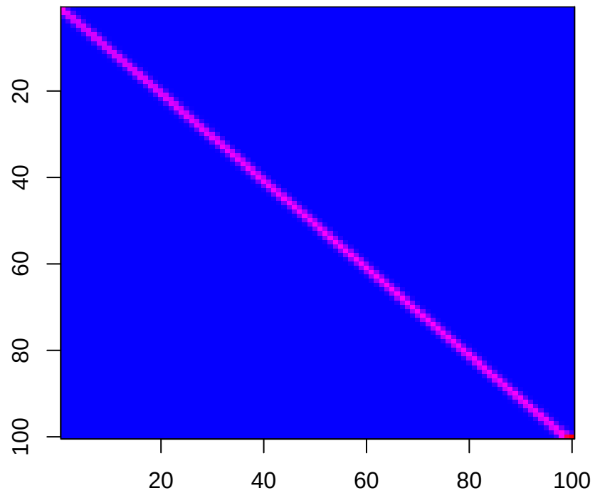
P subkernel
