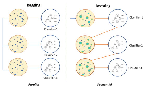
〈Bagging과 Boosting〉
