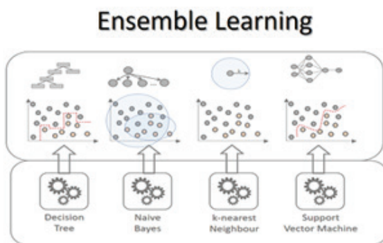
〈앙상블 학습〉
