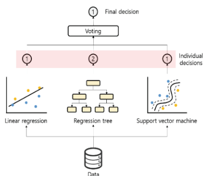
〈Voting〉
