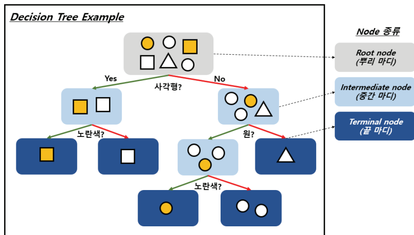
〈의사결정나무 예시〉
