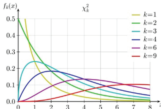
〈카이제곱 그래프〉
