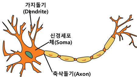
〈신경세포〉
