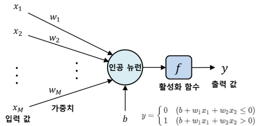
〈퍼셉트론〉
