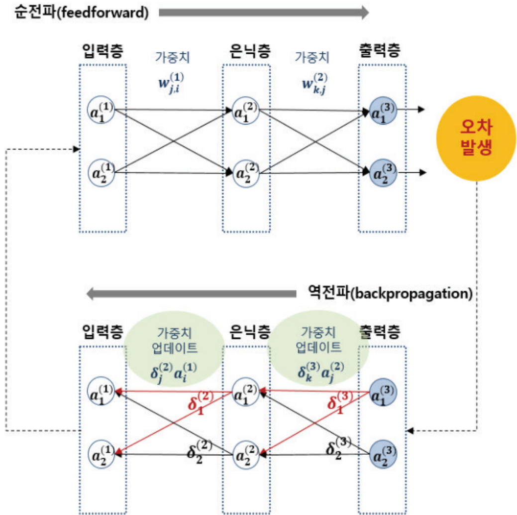
〈순전파(Feedforward)와 역전파(Backpropagation)〉
