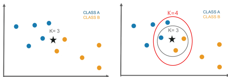
〈K-근접법 예시〉
