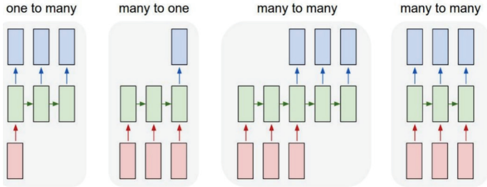
〈순환신경망(RNN)의 유형〉
