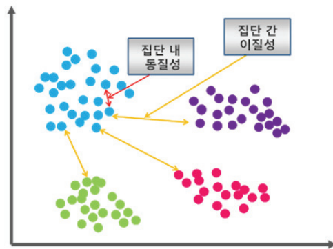
〈군집분석 예시〉
