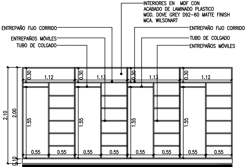
2 INTERIOR SOTANO 1:50
