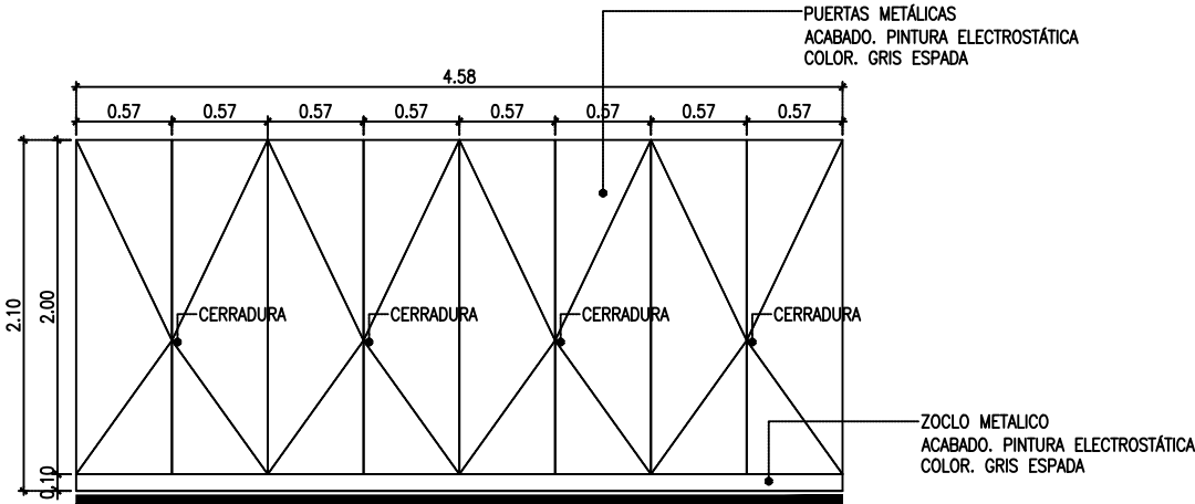
2 ALZADO SOTANO 1:50
