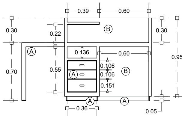
Vista Trasera
