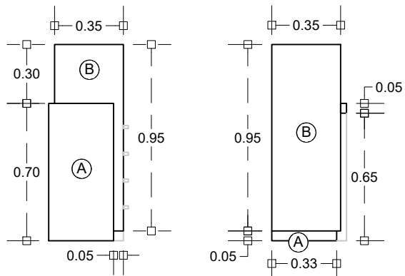
Vista Der.
