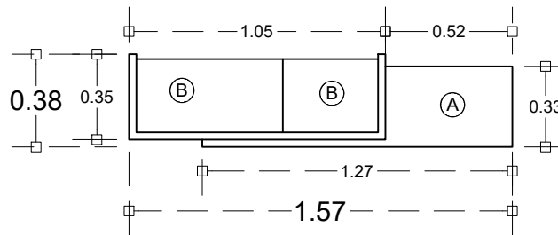
Vista Planta
