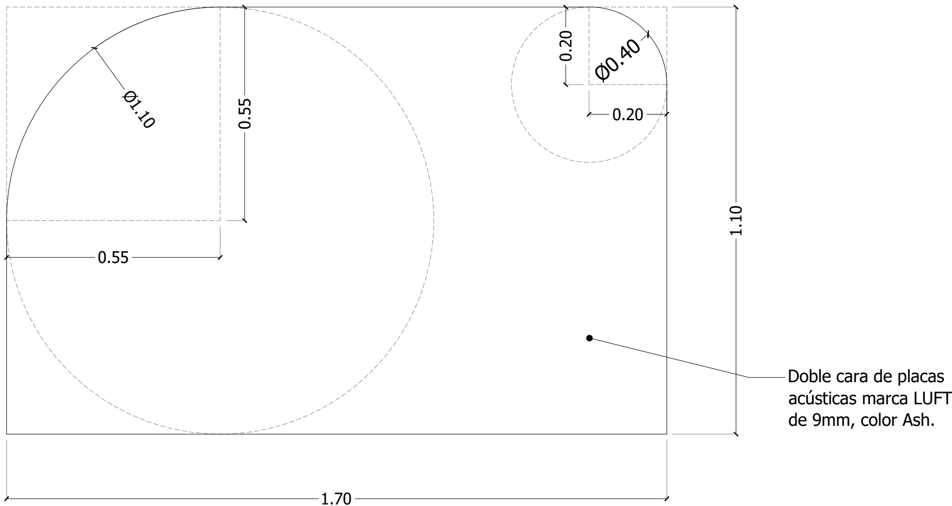
Detalle de Mampara divisoria (corte de acústico) Esc 1:25. Unidades en cm.
