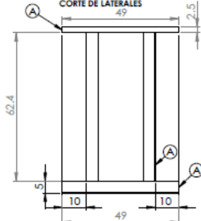
VISTA INFERIOR CORTE DE LATERALES
