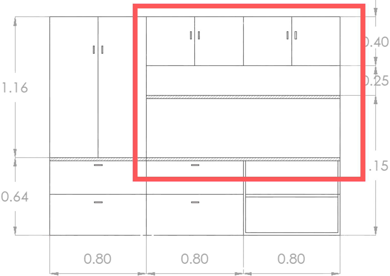
RESPALDO DE 28 MM PARA SOPORTE DE GABIENTE SUPERIOR Y SOPORTE DE REPISA
