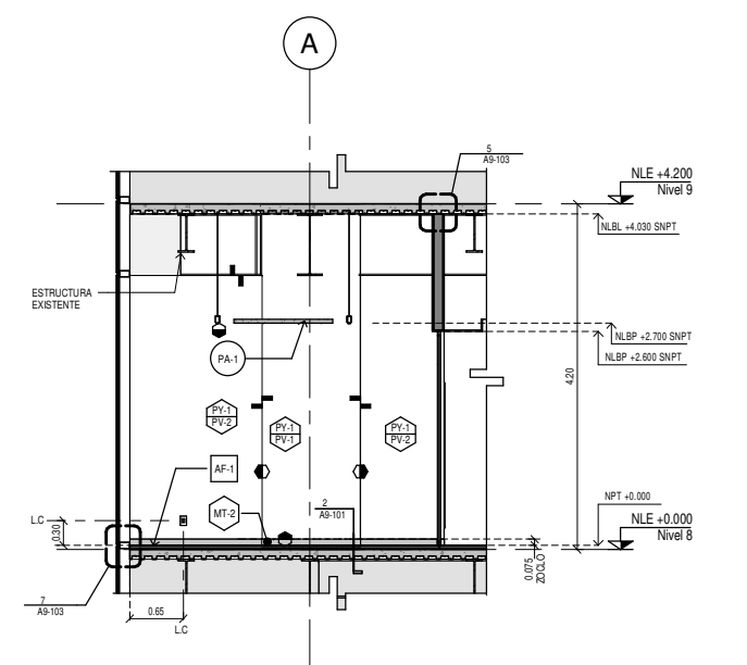
5 Cubículo C. Alzado 02 1 : 50
