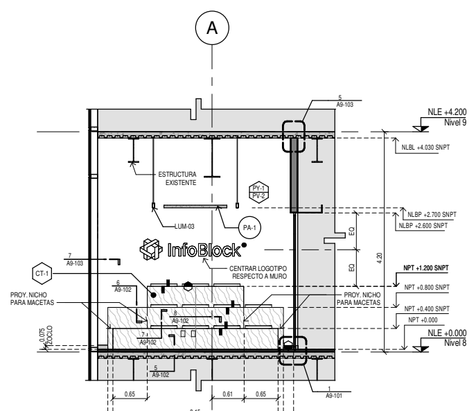
2 Auditorio. Alzado 02 1 : 50
