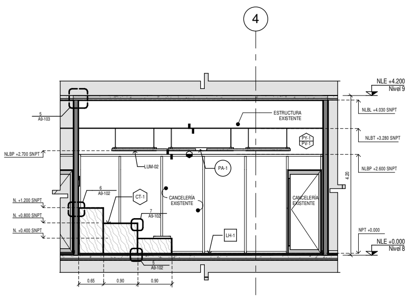
1 Auditorio. Alzado 01 1 : 50
