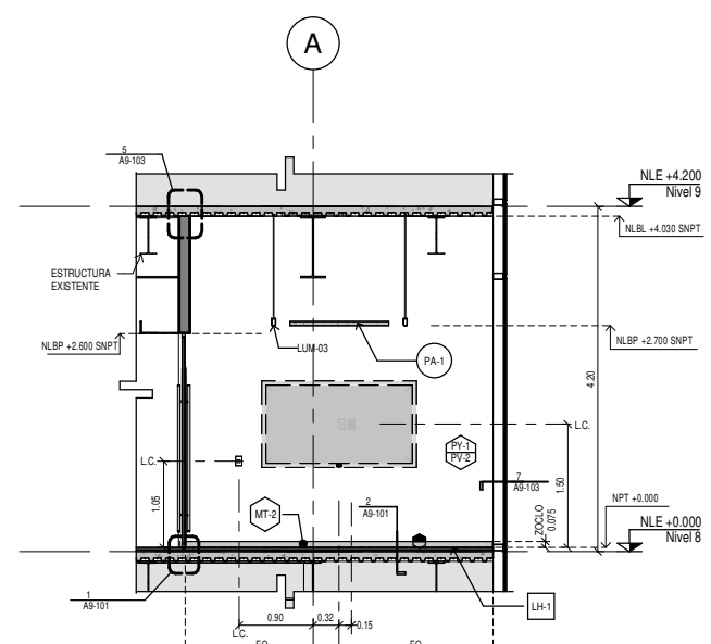
3 Auditorio. Alzado 03 1 : 50
