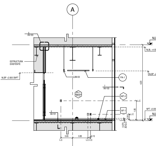
6 Cubículo C. Alzado 03 1 : 50
