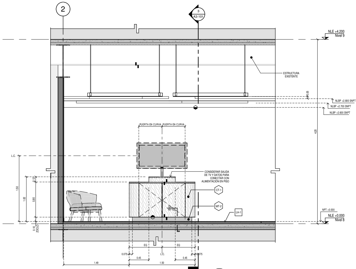
4 Mamparas Demostración. Alzado frontal. 1 : 25
