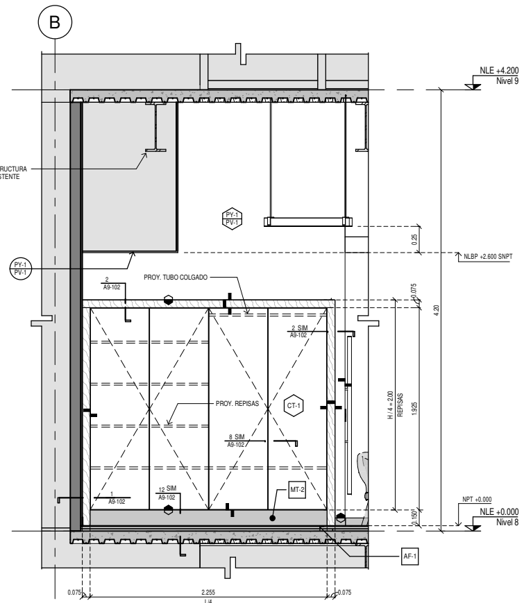
3 Clóset. Alzado Parcial 01 1 : 25
