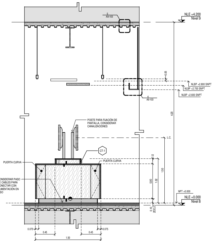
5 Mamparas Demostración. Alzado lateral.
