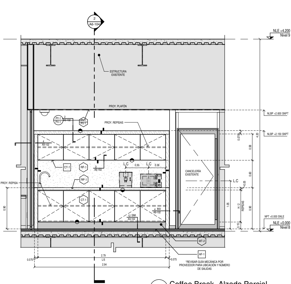
1 Coffee Break. Alzado Parcial 1 : 25
