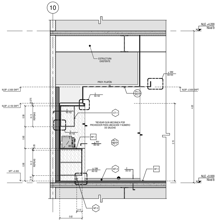
2 Coffee Break. Alzado Parcial 02 1 : 25
