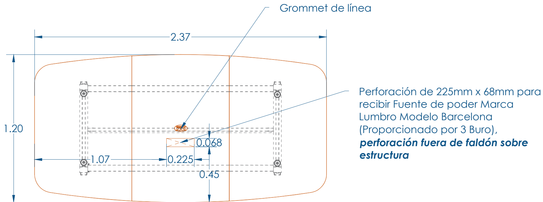
Vista superior
