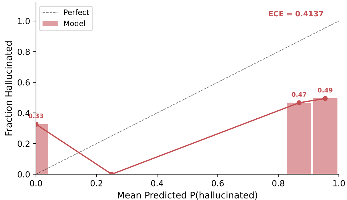
Phi-3-Vision-4B ⚠
