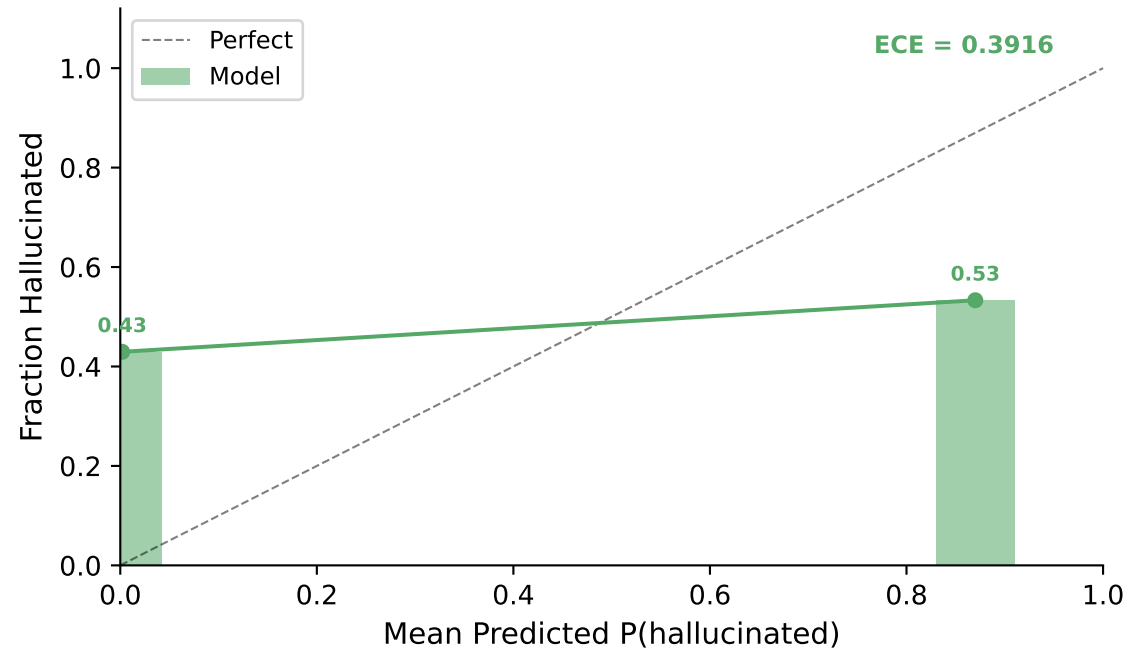
LLaVA-1.5-13B ⚠
