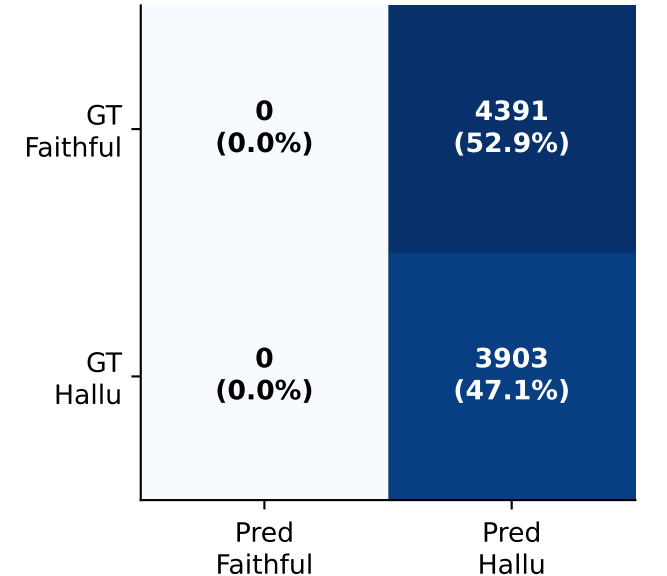
LLaVA-1.5-13B
