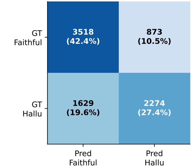
MedGemma-27B
