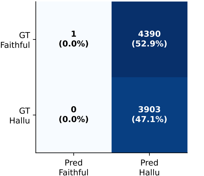
Phi-3-Vision-4B
