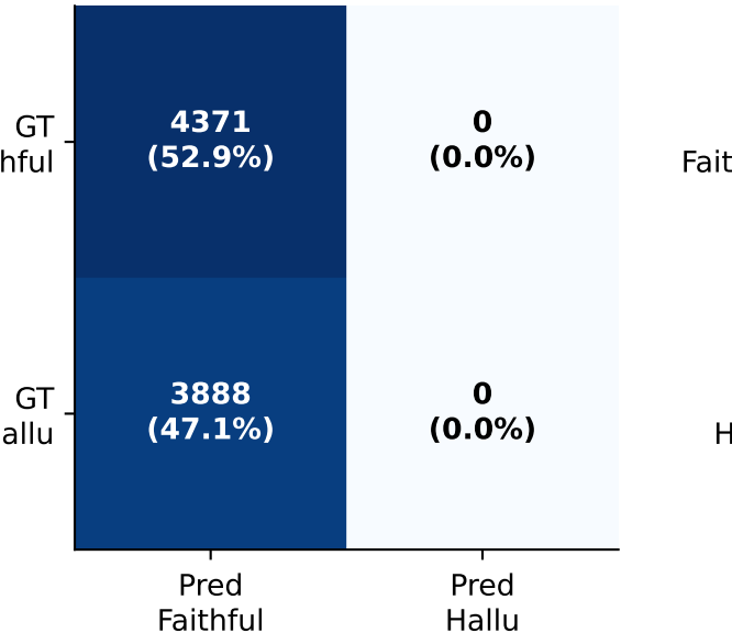
BioViL-T
