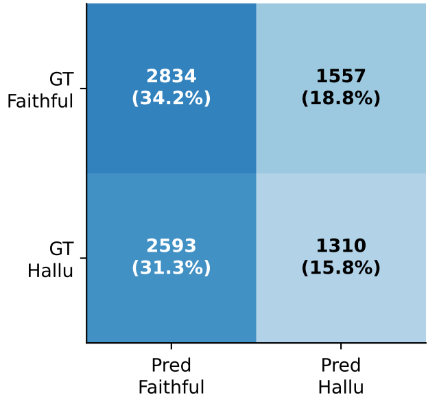
BLIP-2-OPT-6.7B
