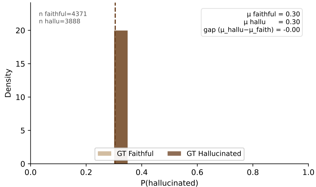
BioViL-T
