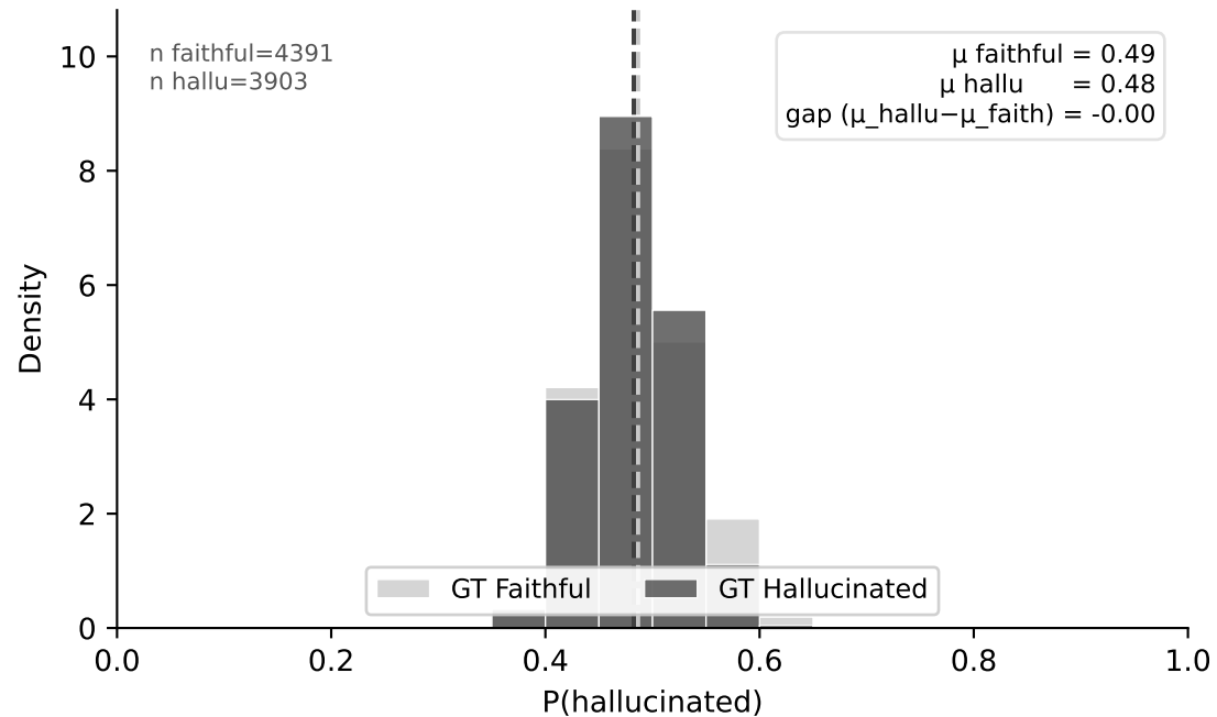
BLIP-2-OPT-6.7B
