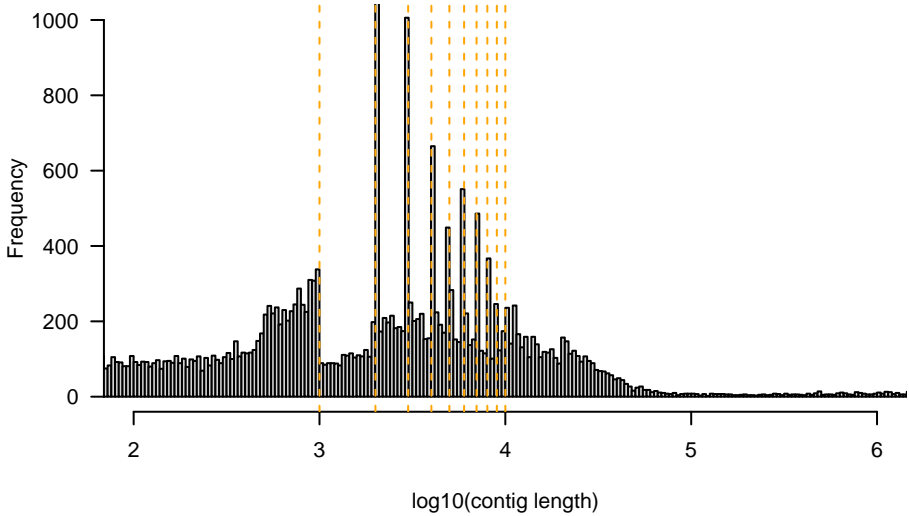
Histogram of \log_{10}(d)
