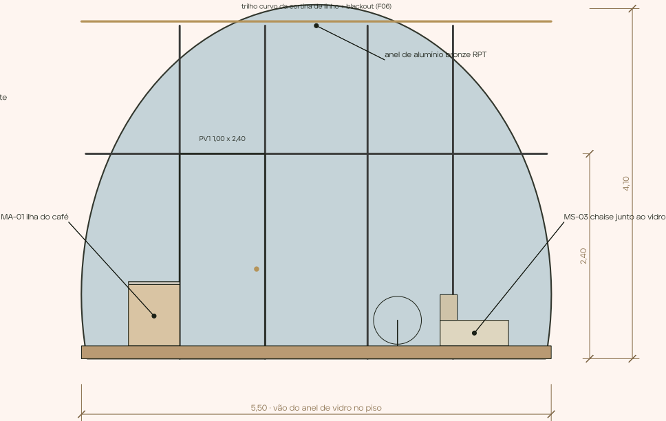
ELEVAÇÃO D · FACHADA INTERNA · x = 0,90
