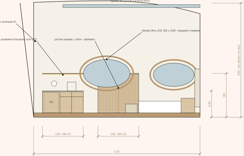
ELEVAÇÃO B · LATERAL ESQUERDA · y = +2,90
