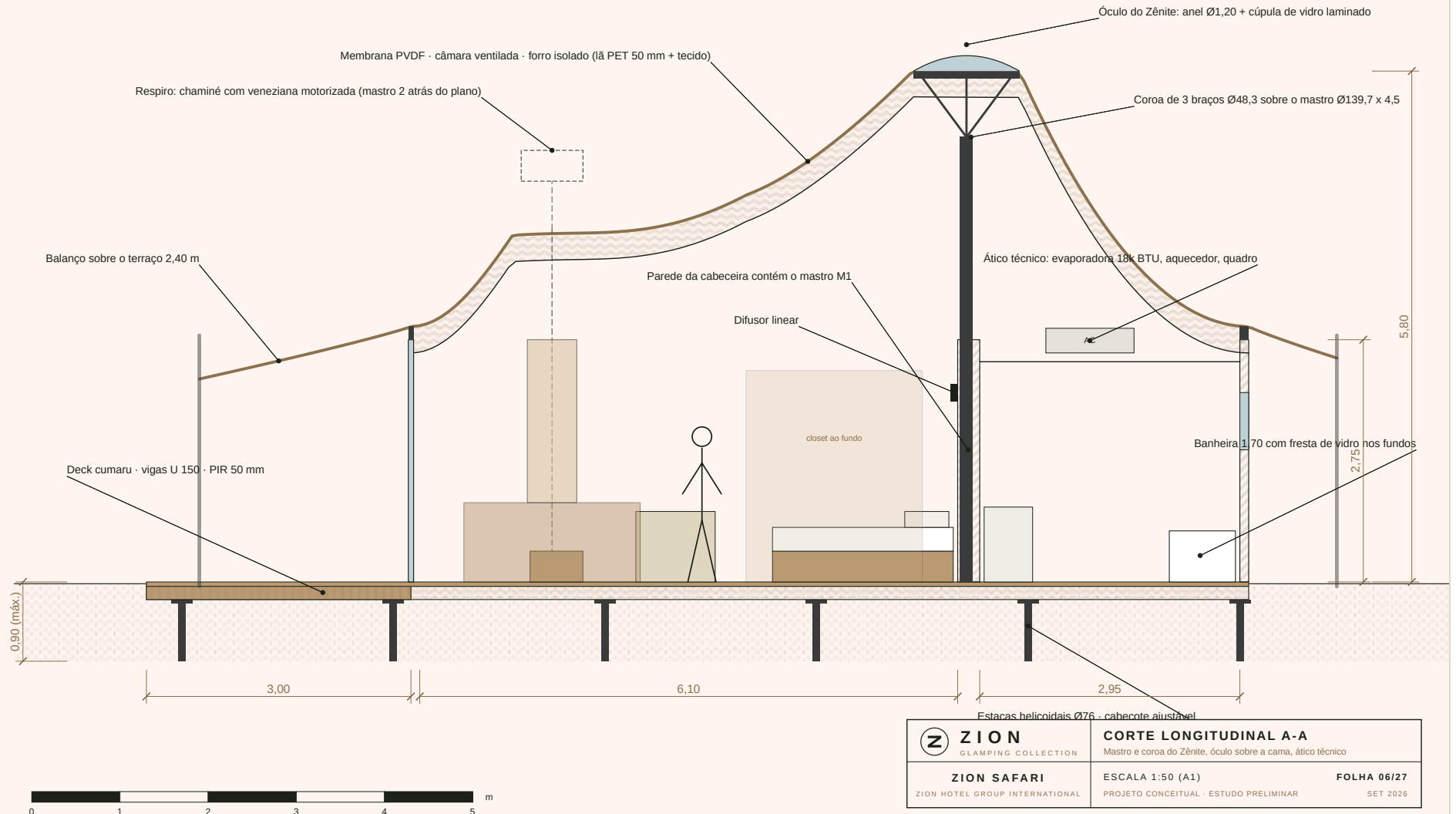
CORTE LONGITUDINAL
