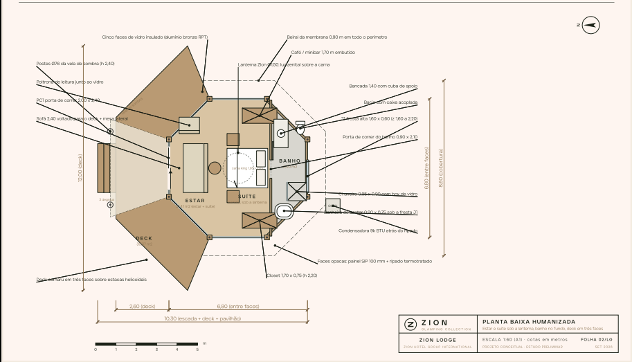
Planta humanizada · sem escala nesta página
