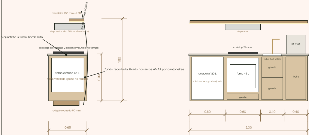
MA-01 · MINI COZINHA · CORTE 1:20 (módulo forno + cooktop) MA-01 · MINI COZINHA · VISTA FRONTAL 1:20
