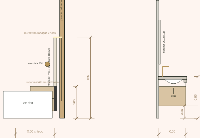
MA-03 · CABECEIRA E CRIADO SUSPENSO · CORTE 1:15 MA-04 · BANCADA · CORTE 1:15
