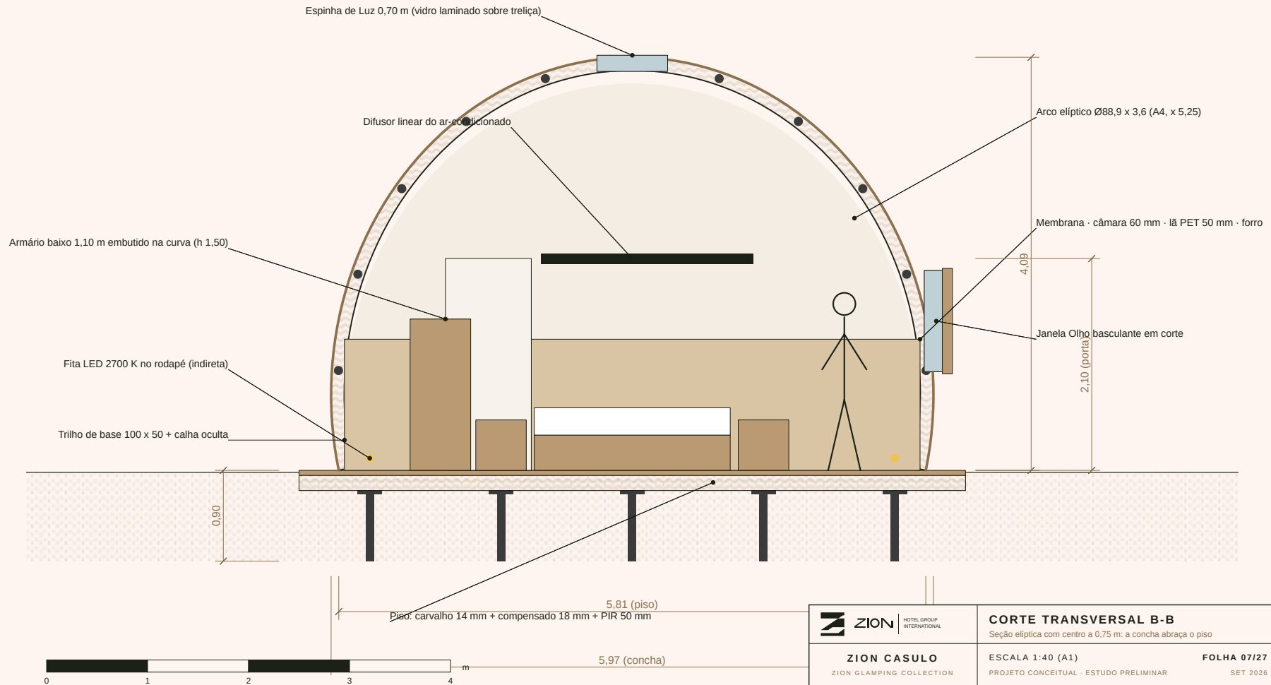
CORTE TRANSVERSAL
