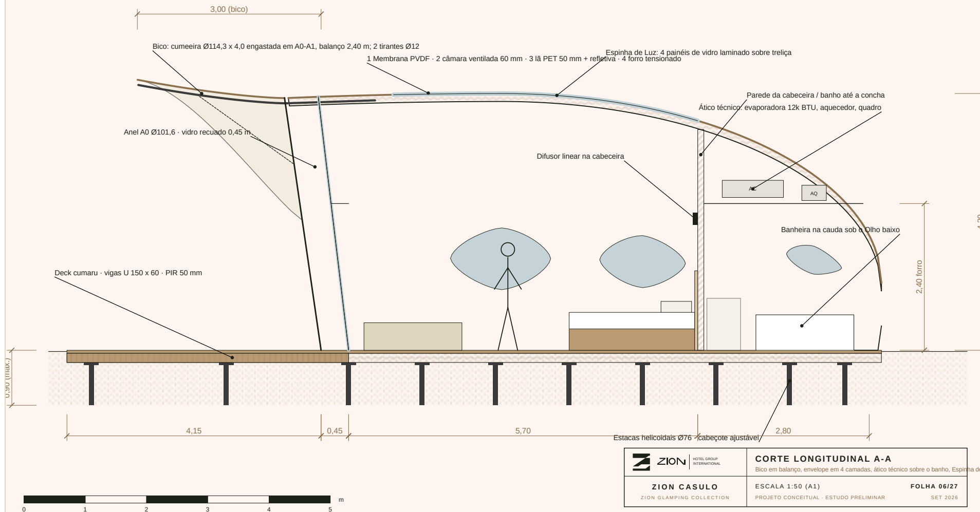
CORTE LONGITUDINAL
