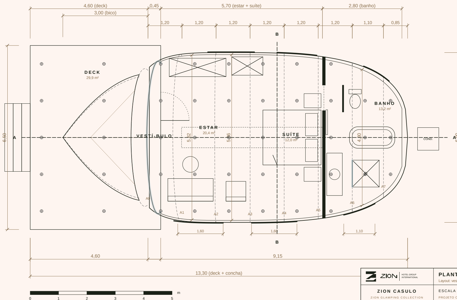
PLANTA BAIXA COTADA
