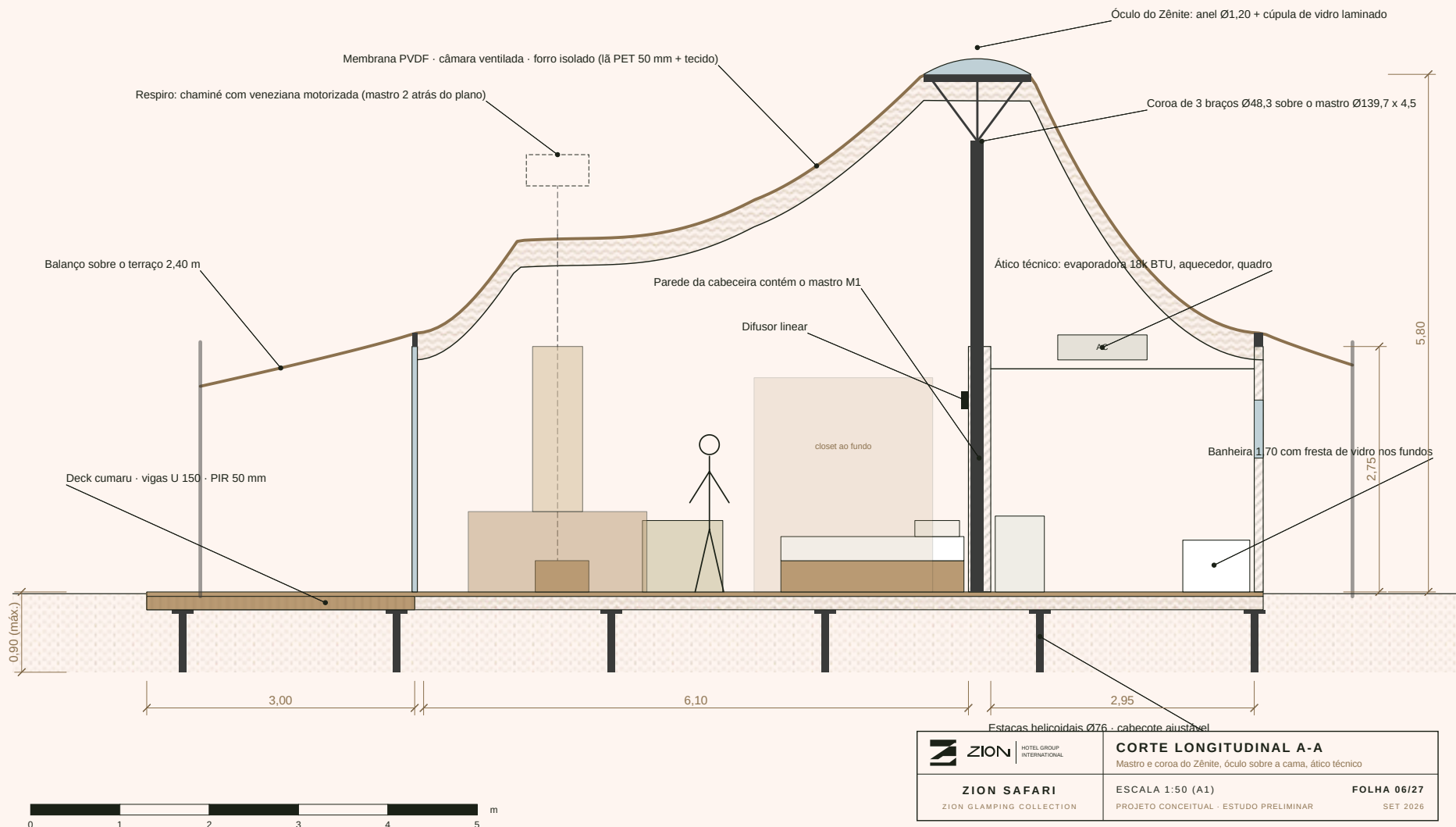
CORTE LONGITUDINAL
