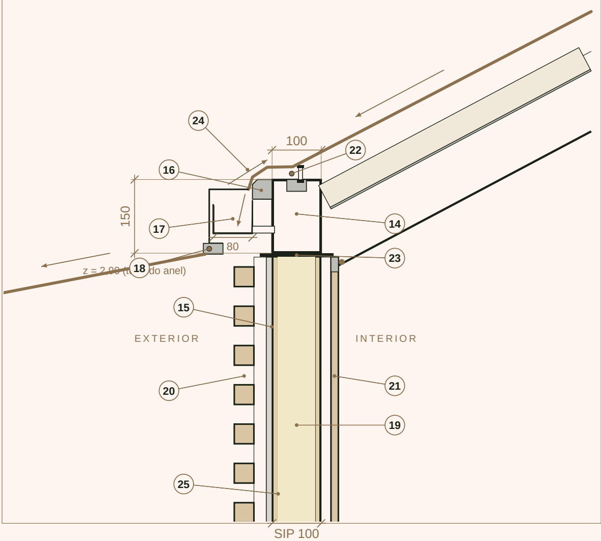
SEÇÃO B - ANEL DE BEIRAL SOBRE PILAR
