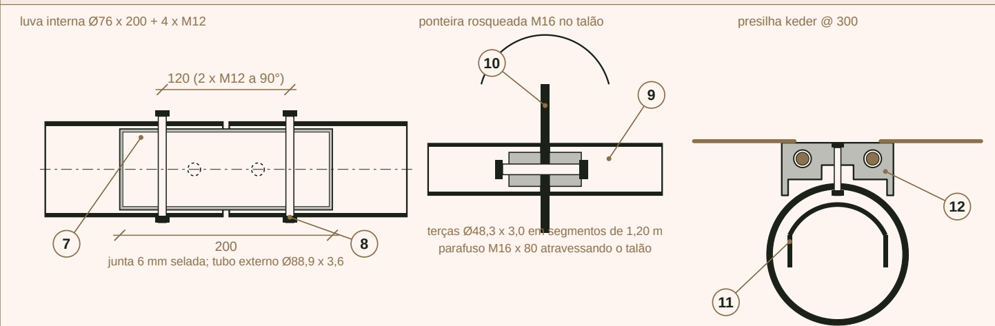
1:60 / sem escala
