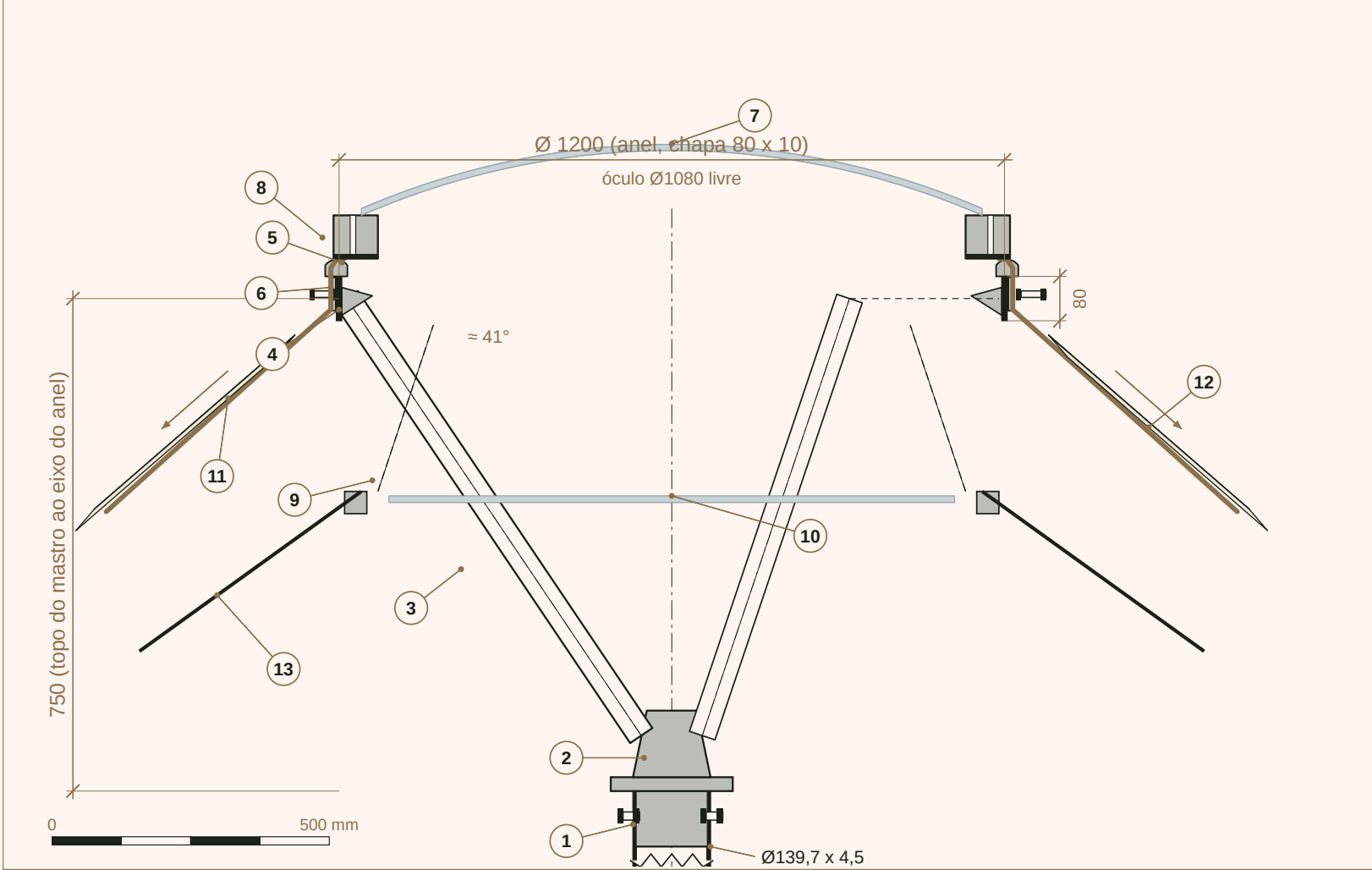
SEÇÃO A - ANEL DO ZÊNITE Ø1200 COM ÓCULO DE VIDRO
