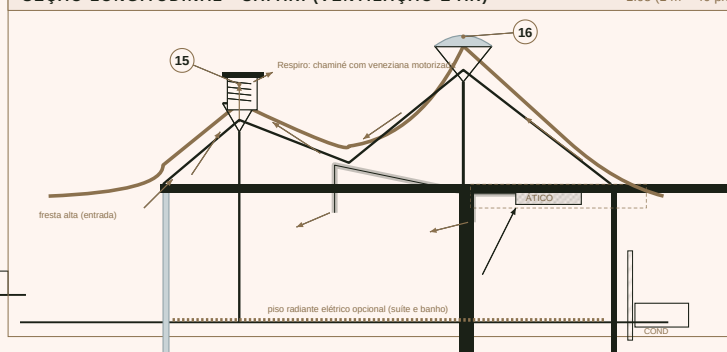
SEÇÃO LONGITUDINAL - SAFARI (VENTILAÇÃO E AR) ≈ 1:95 (1 m = 40 px)
