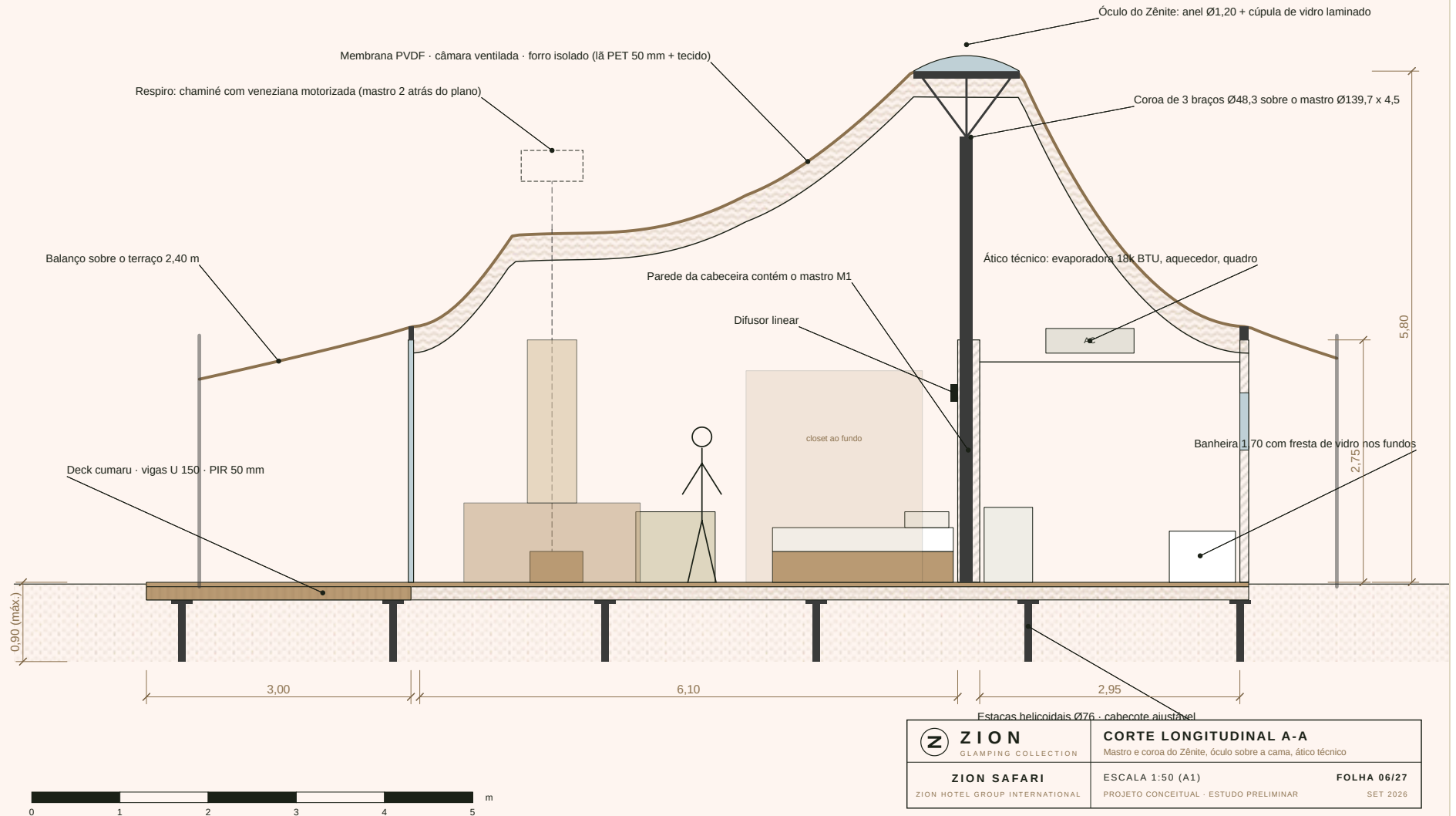
CORTE LONGITUDINAL
