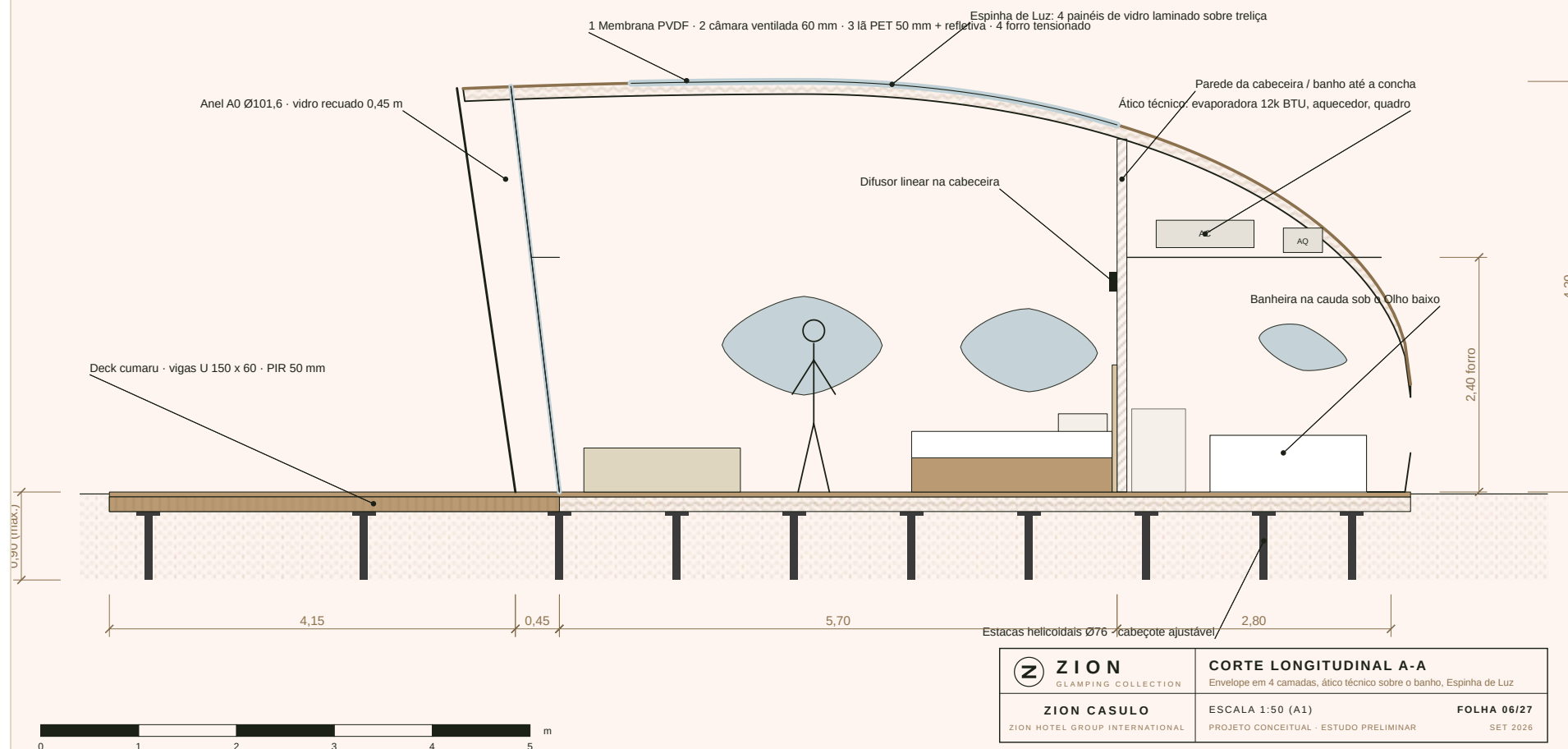
CORTE LONGITUDINAL
