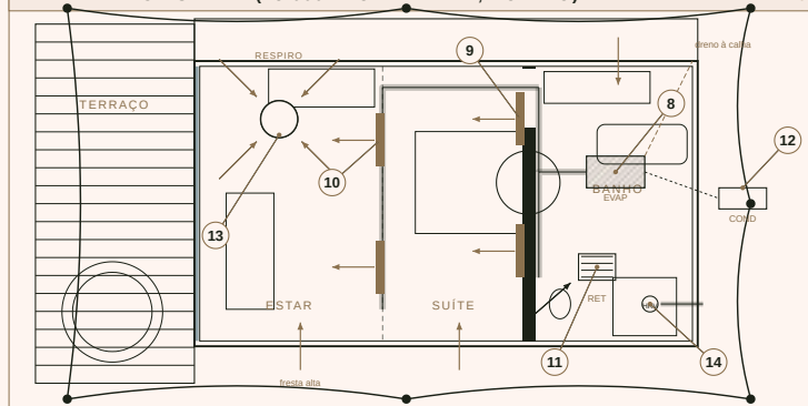
PLANTA - ZION SAFARI (18.000 BTU INVERTER, DUTADO) 1:100
