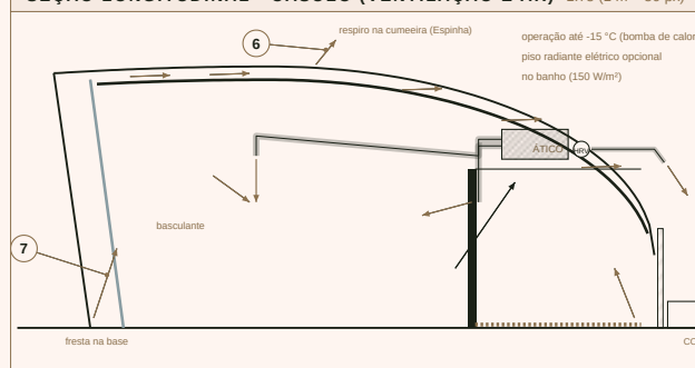
SEÇÃO LONGITUDINAL - CASULO (VENTILAÇÃO E AR) 1:75 (1 m = 50 px)
