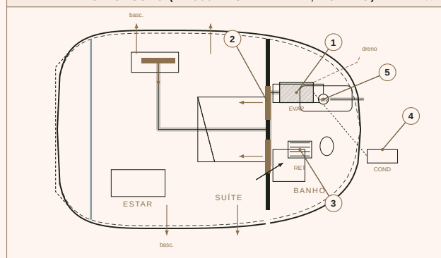
PLANTA - ZION CASULO (12.000 BTU INVERTER, DUTADO) 1:100
