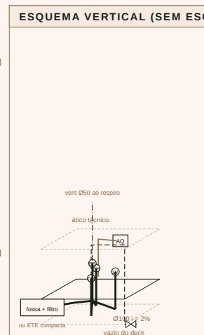
ESQUEMA VERTICAL (SEM ESCALA)
