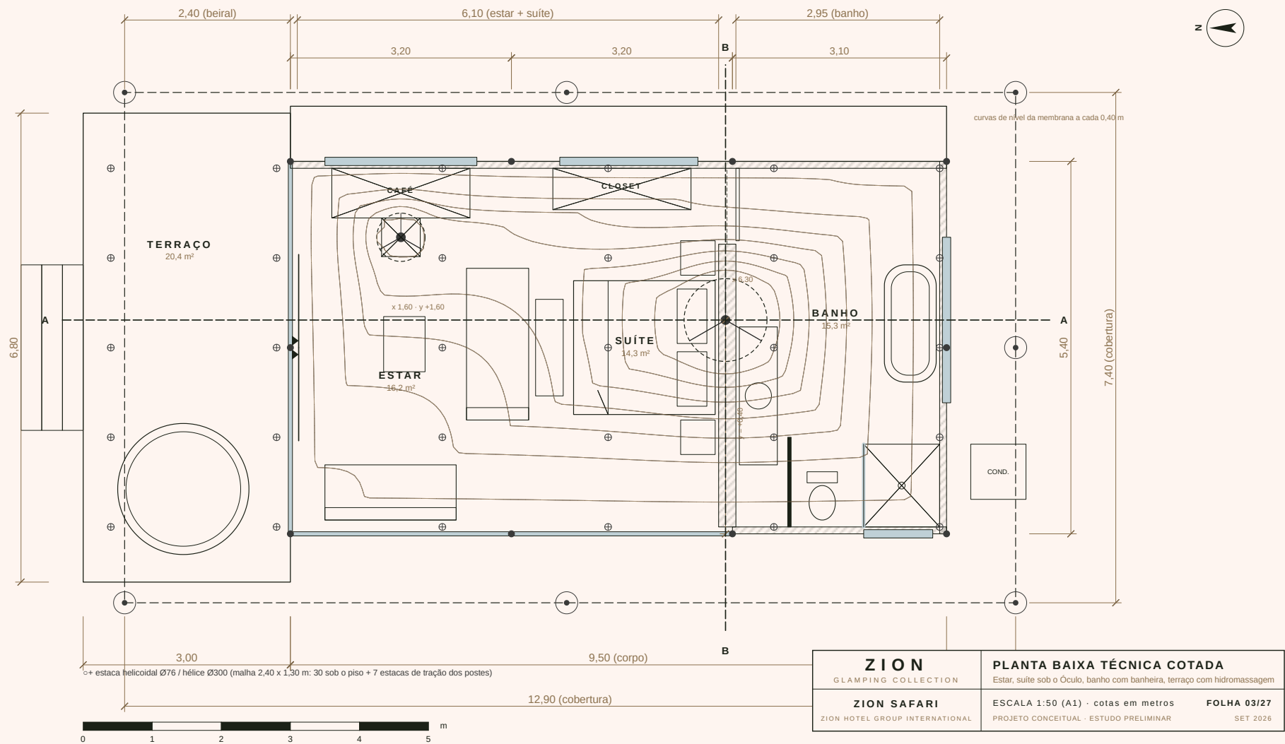
PLANTA BAIXA COTADA
