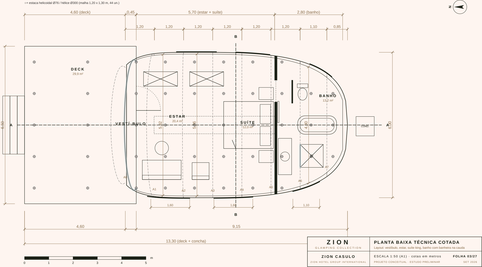
PLANTA BAIXA COTADA
