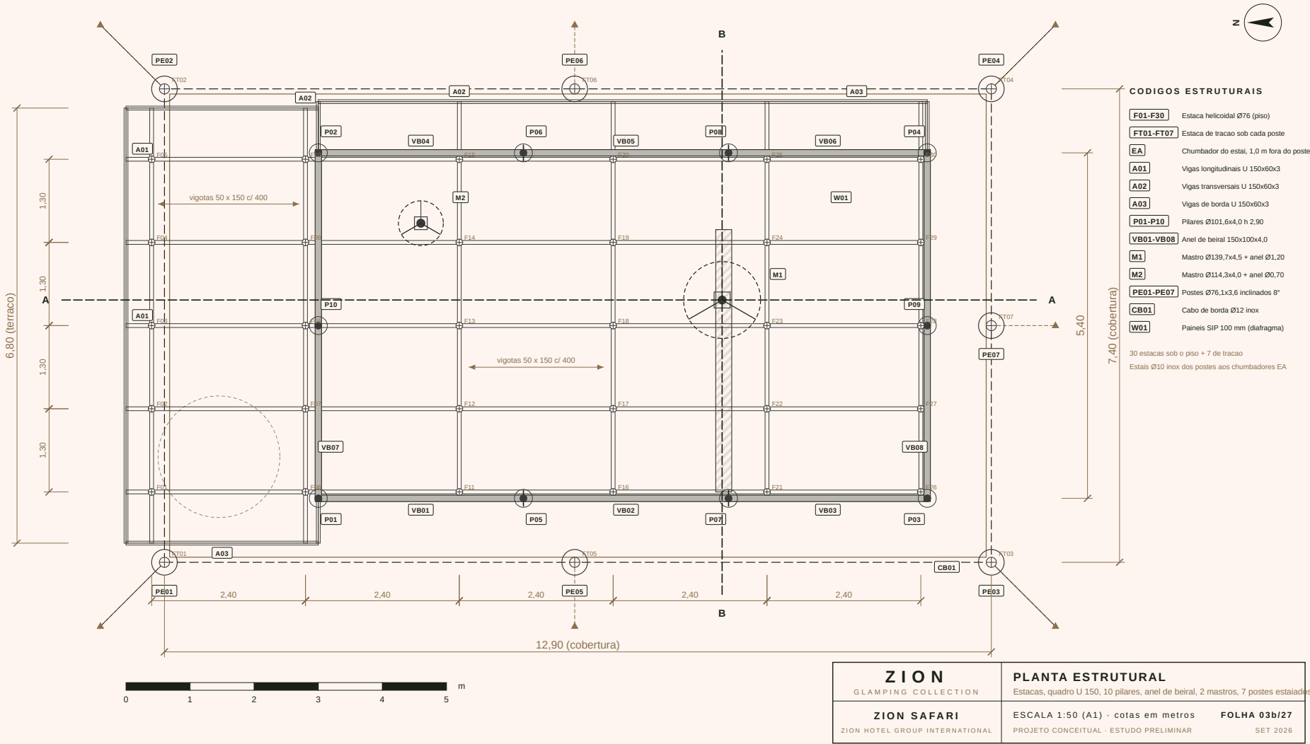
PLANTA ESTRUTURAL
