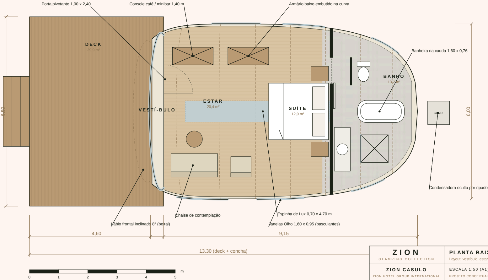
PLANTA DE LAYOUT
