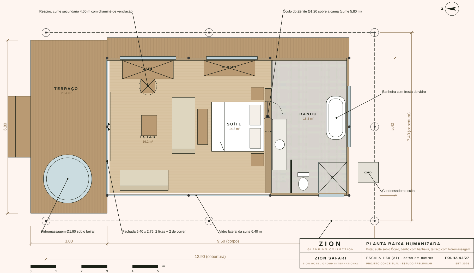
PLANTA DE LAYOUT
