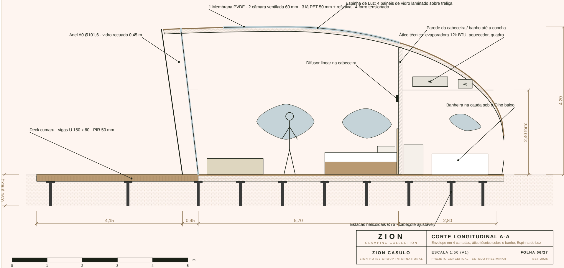
CORTE LONGITUDINAL
