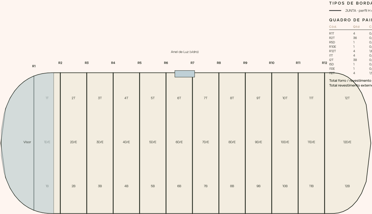
Vista lateral · painéis de ACM entre anéis em 4 setores (T topo, D/E lados, B barriga) · juntas em perfil H · revestimento interno em compensado curvado
