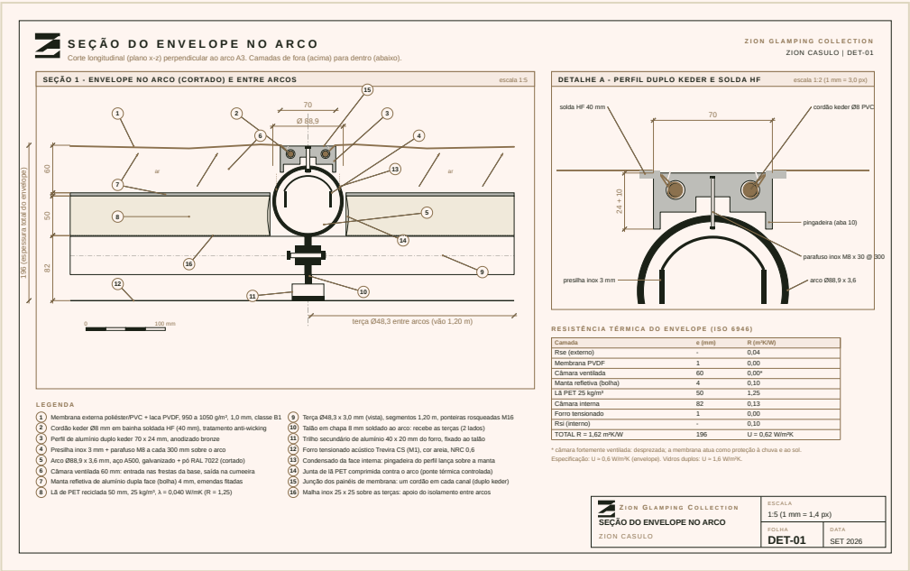
DET-01: seção do envelope no arco, resistência térmica U ≈ 0,62 W/m2K (envelope) · vidro U ≈ 1,6 W/m2K.
