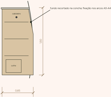
MA-02 · ARMÁRIO ACOPLADO À CURVA · CORTE 1:20
