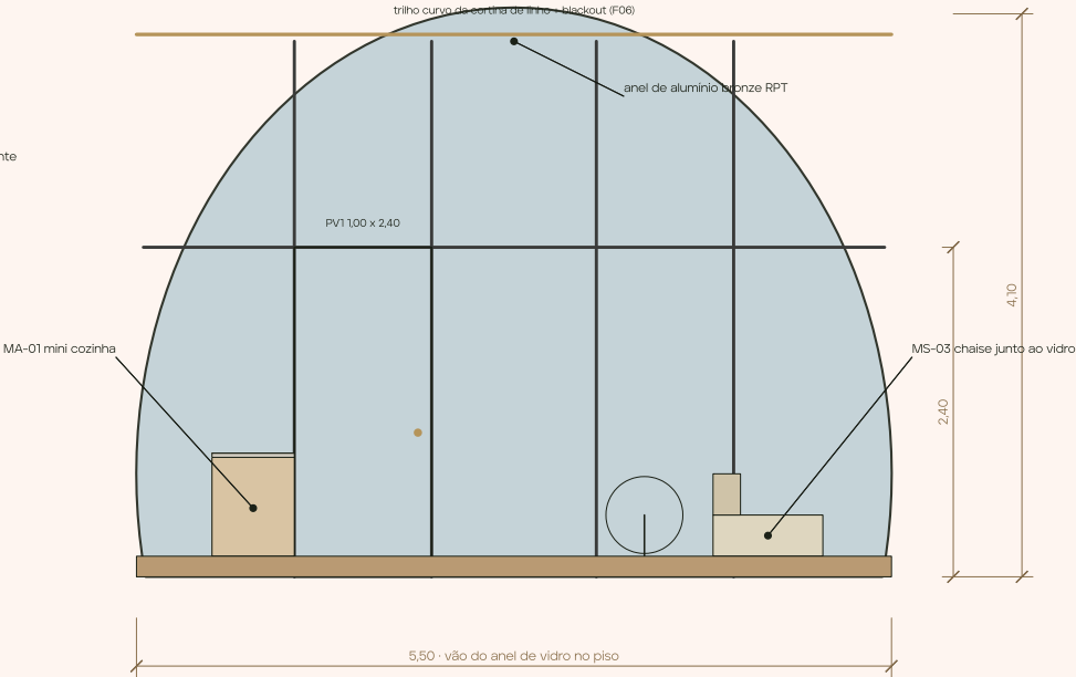
ELEVAÇÃO D · FACHADA INTERNA · x = 0,90
