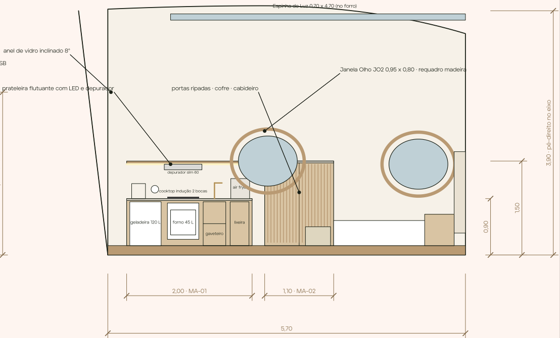
ELEVAÇÃO B · LATERAL ESQUERDA · y = +2,90
