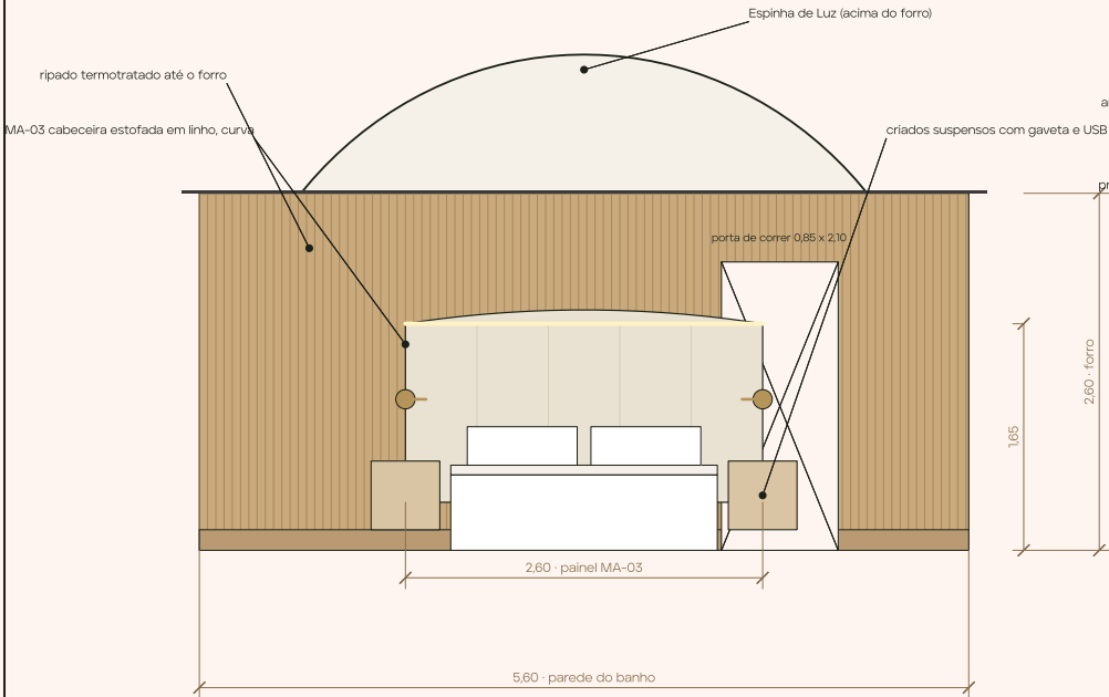
ELEVAÇÃO A · CABECEIRA · x = 6,60
