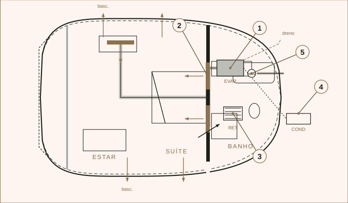
PLANTA - ZION CASULO (12.000 BTU INVERTER, DUTADO)
