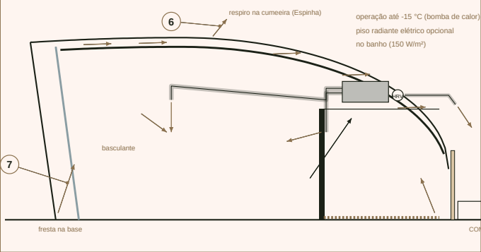
SEÇÃO LONGITUDINAL - CASULO (VENTILAÇÃO E AR)
