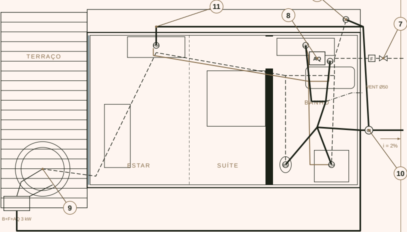
PLANTA HIDRÁULICA - ZION SAFARI
