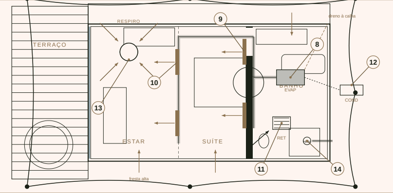
PLANTA - ZION SAFARI (18.000 BTU INVERTER, DUTADO)
