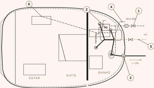
PLANTA HIDRÁULICA - ZION CASULO
