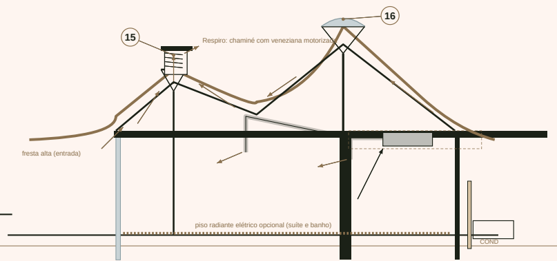
SEÇÃO LONGITUDINAL - SAFARI (VENTILAÇÃO E AR)
