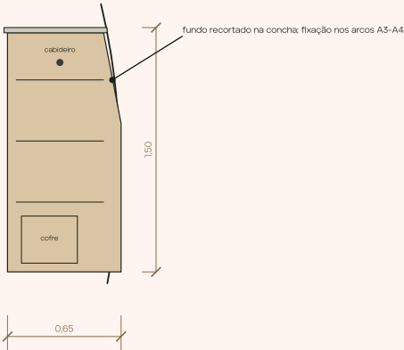
MA-02 · ARMÁRIO ACOPLADO À CURVA · CORTE 1:20
