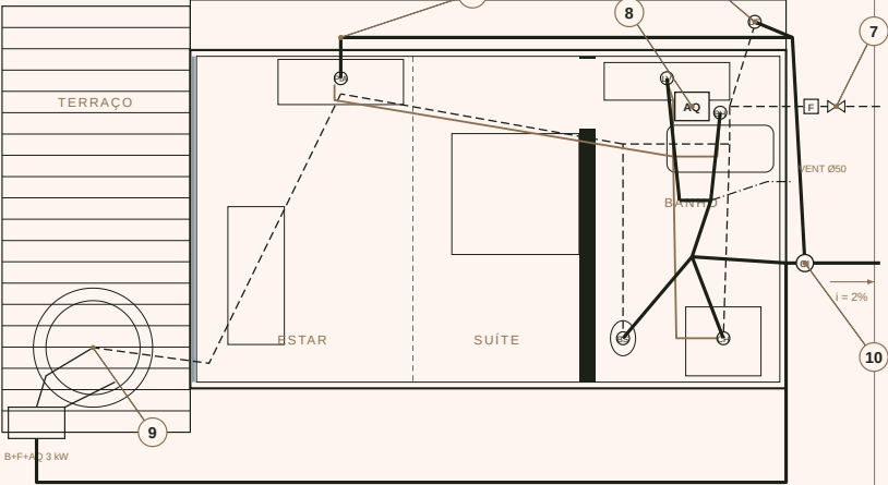
PLANTA HIDRÁULICA - ZION SAFARI
