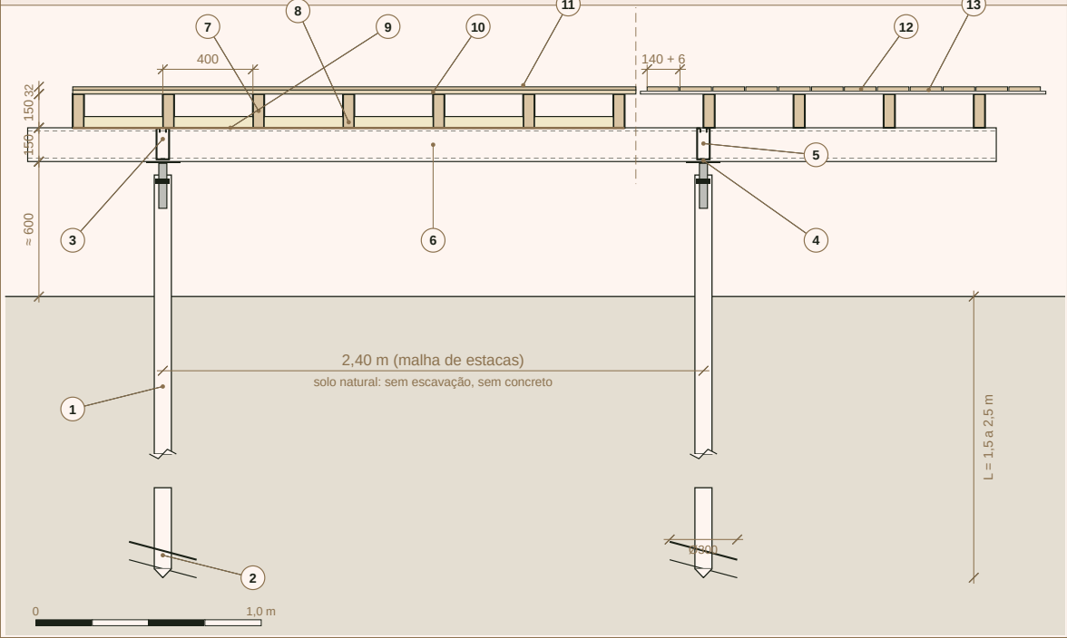
SEÇÃO TRANSVERSAL DO DECK - TERRENO PLANO
