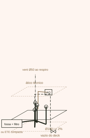
ESQUEMA VERTICAL (SEM ESCALA)
