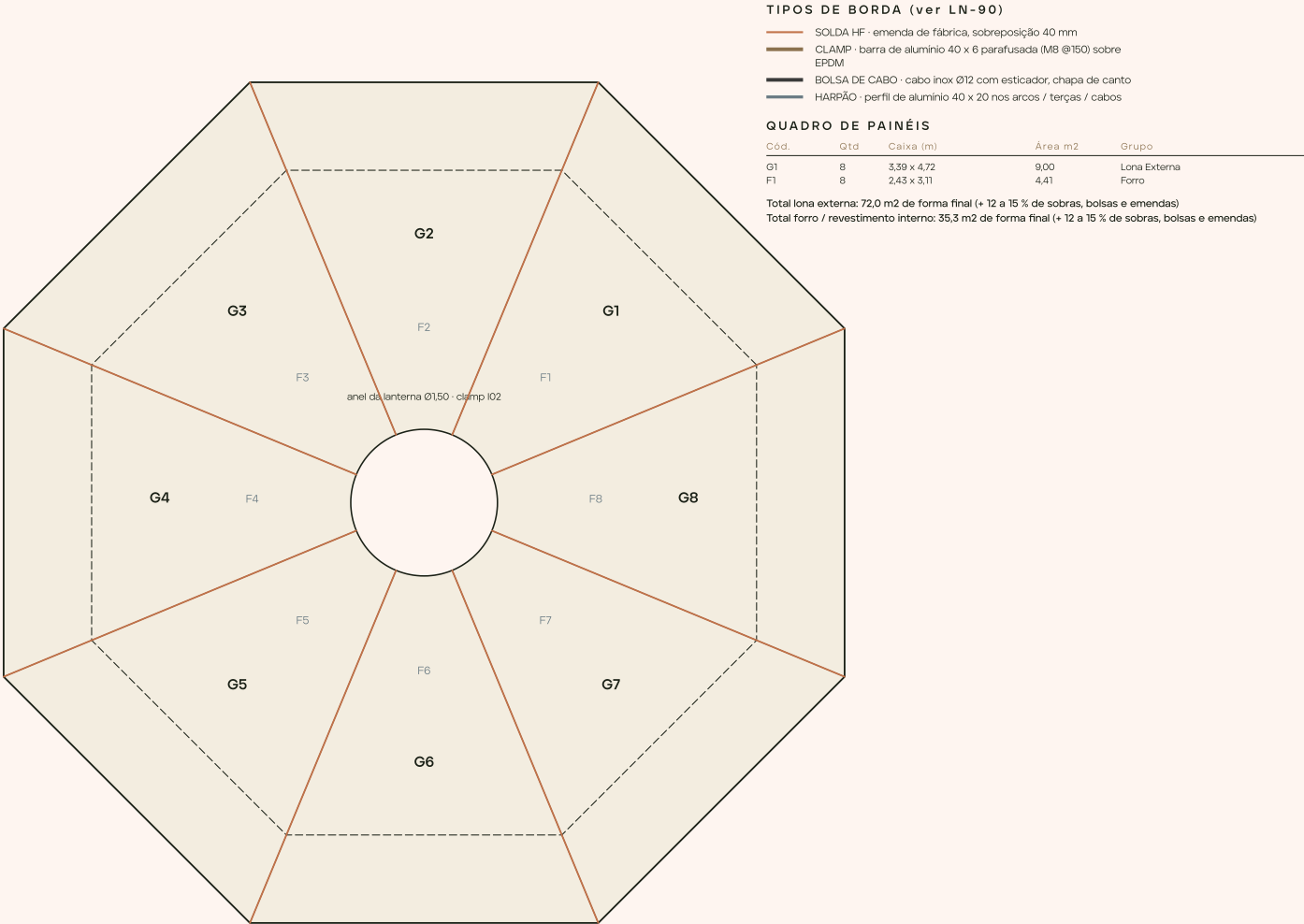
Planta da cobertura - 8 gomos iguais soldados sobre os caibros - bolsa de cabo no beiral (perfil I01) - forro em
