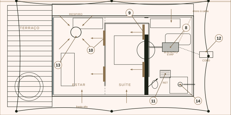
PLANTA - ZION SAFARI (18.000 BTU INVERTER, DUTADO)
