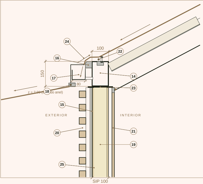
SEÇÃO B - ANEL DE BEIRAL SOBRE PILAR
