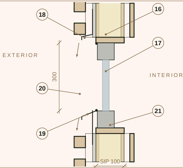
(D) FRESTA DE VIDRO NO PAINEL SIP 100 COM RUFOS
