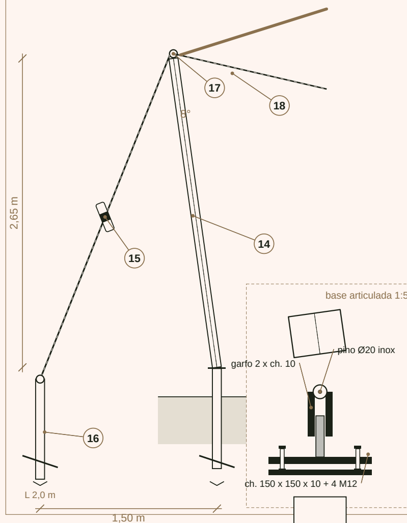
(B) POSTE EXTERNO SAFARI: BASE E ESTAI
