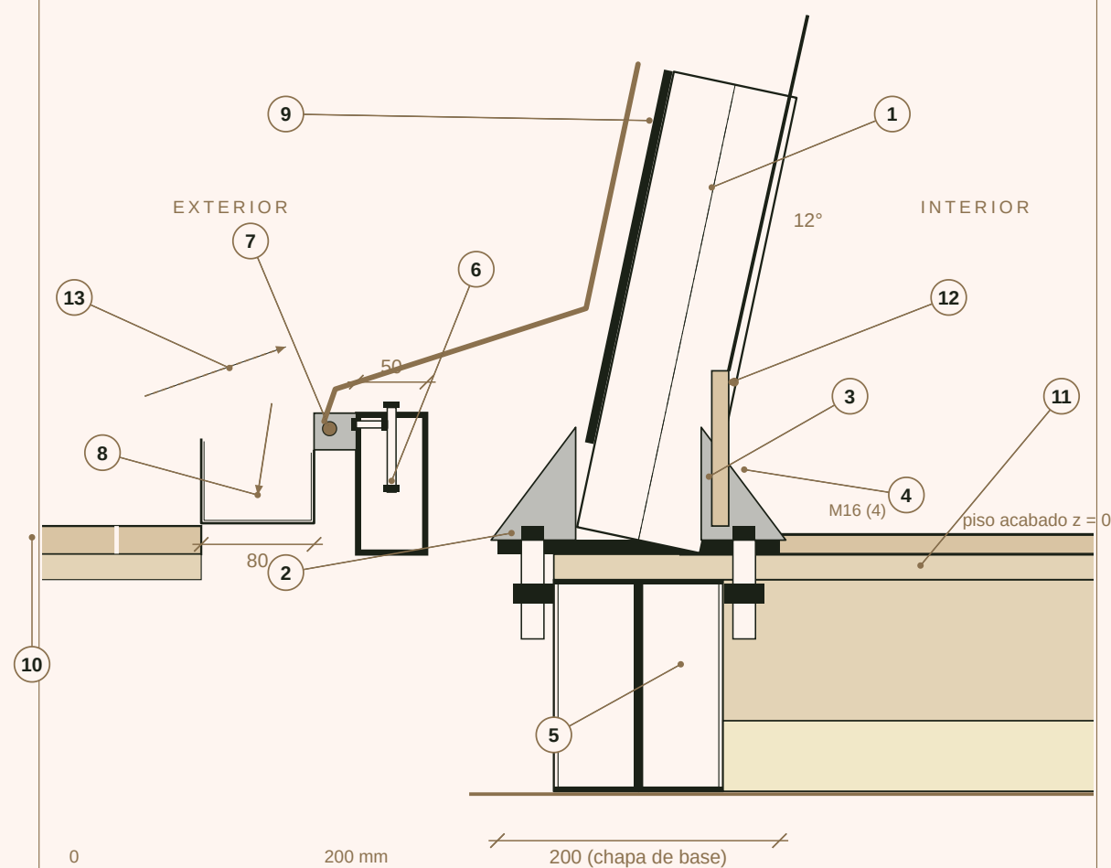
(A) PÉ DE ARCO CASULO SOBRE VIGA DE BORDA
