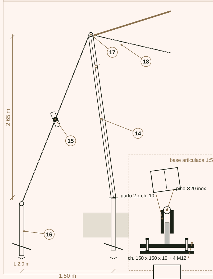
(B) POSTE EXTERNO SAFARI: BASE E ESTAI
