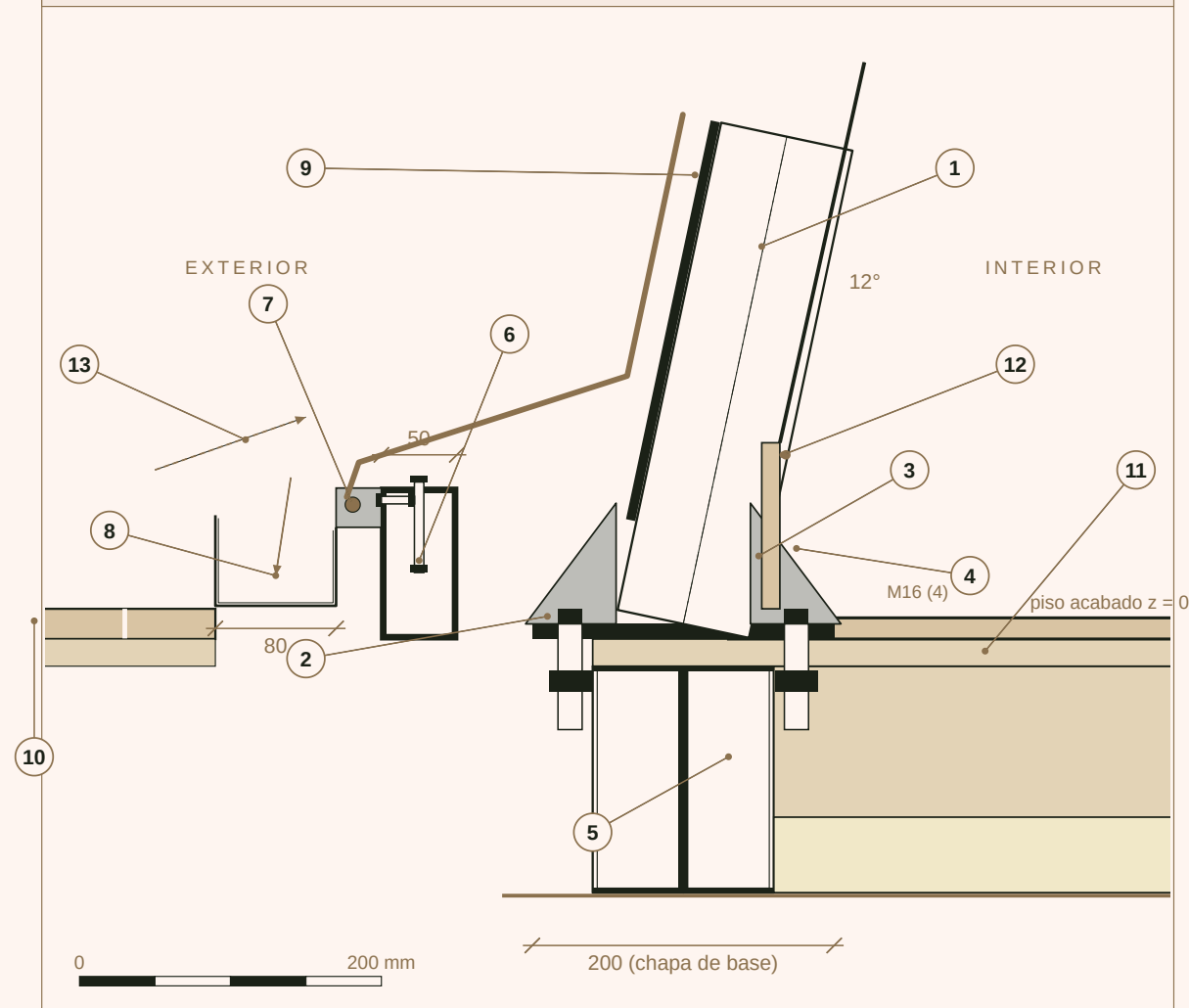
(A) PÉ DE ARCO CASULO SOBRE VIGA DE BORDA
