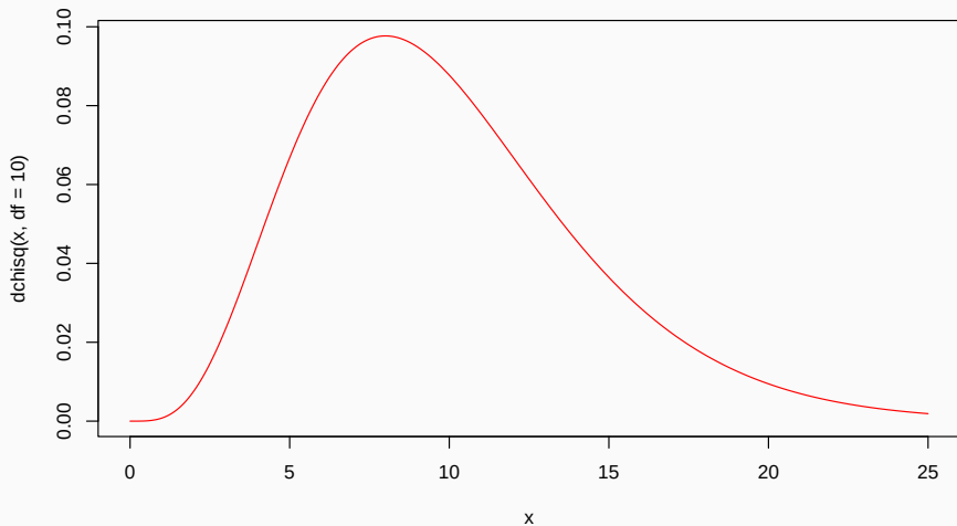
Chi-Quadrat-Verteilung
