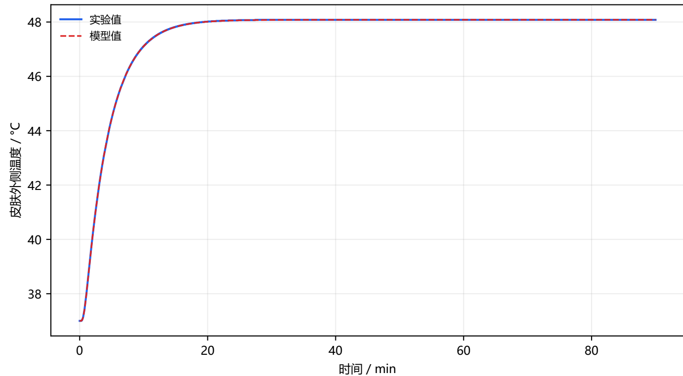
问题一：模型拟合结果
