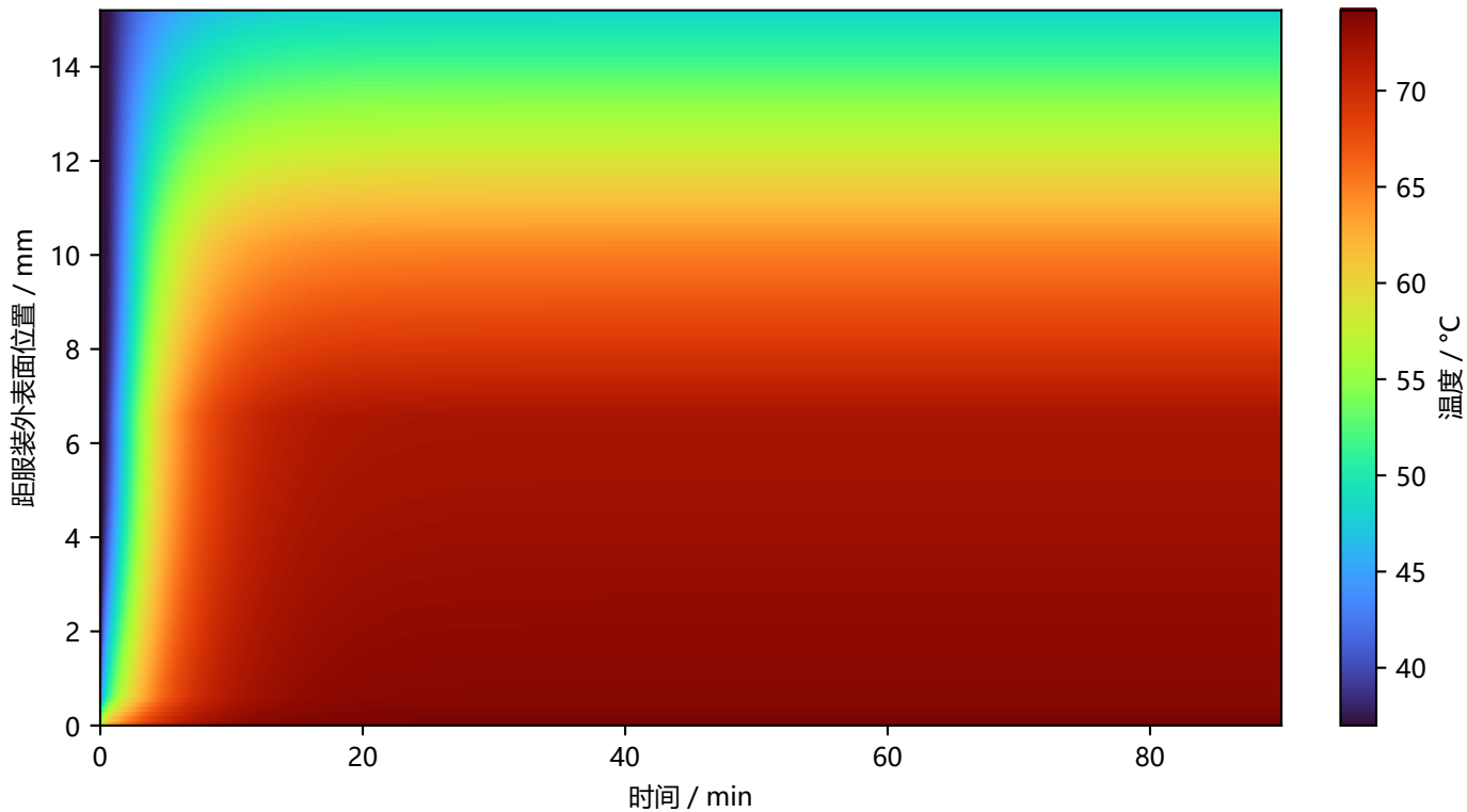
四层介质温度场
