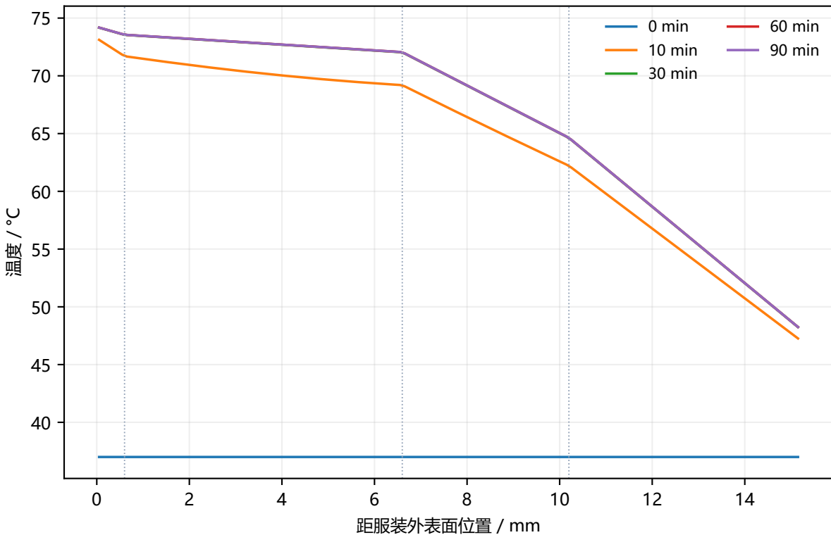
典型时刻温度剖面
