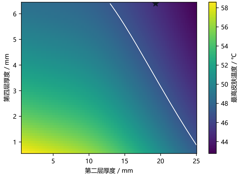
最高温度响应面与 47°C 边界
