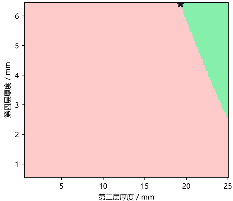
离散可行域 (绿)
