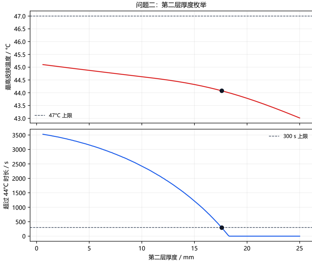
图 7 问题二第二层厚度枚举及安全约束
