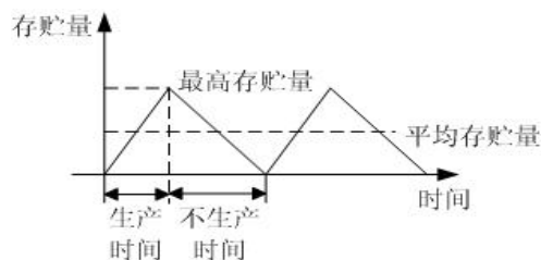
图 4 经济生产批量模型存贮量的变化情况
