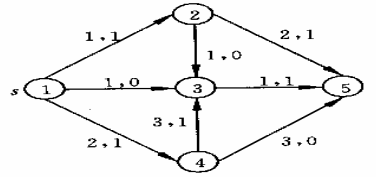
图 6 最大流问题
