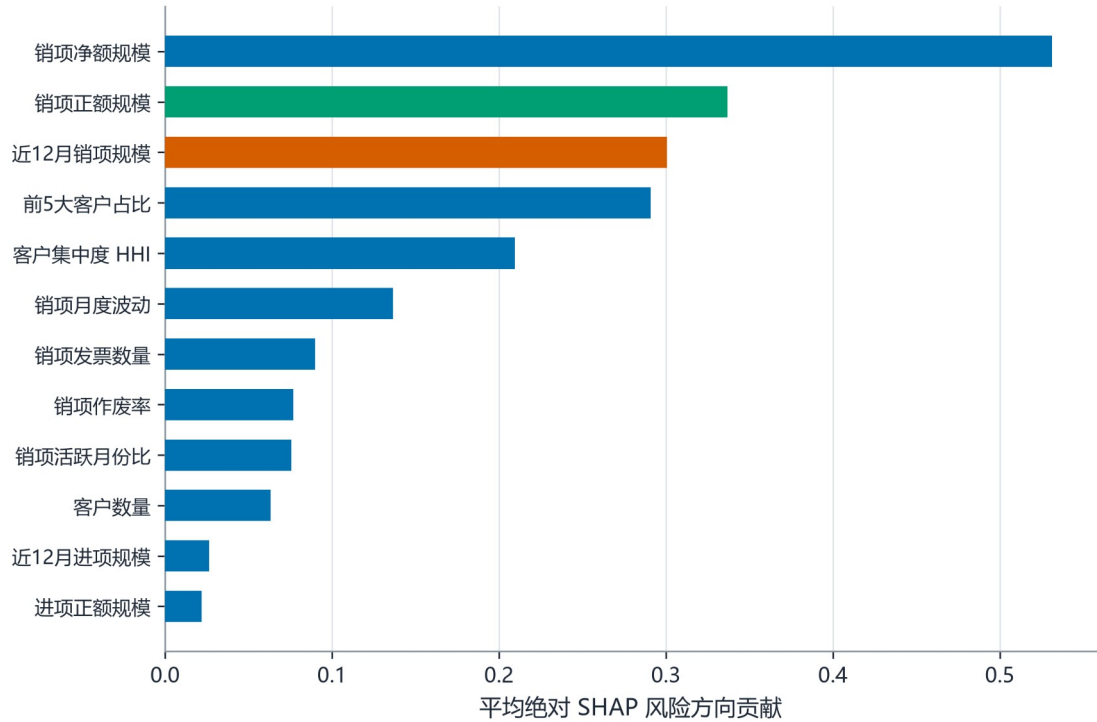
图 10 XGBoost 分量的全局 SHAP 风险方向重要性（纵轴保留模型原始特征名，横轴为平均绝对 SHAP 风险方向贡献）
