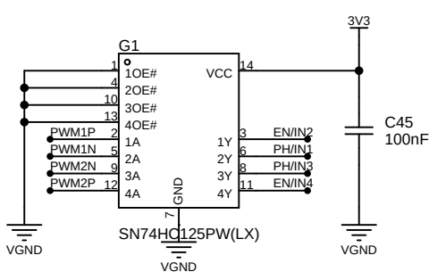
四路缓冲器
