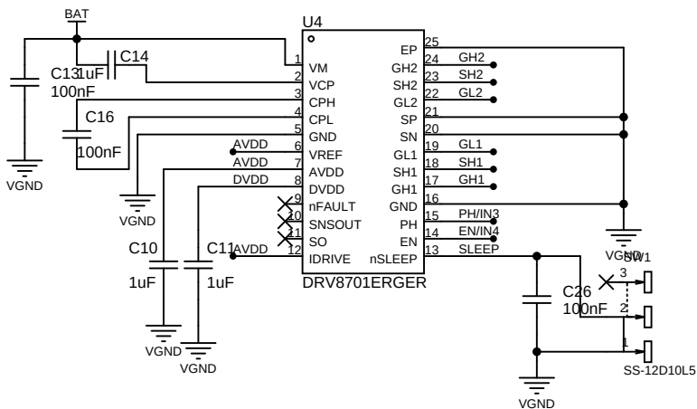
栅极驱动 & H桥
