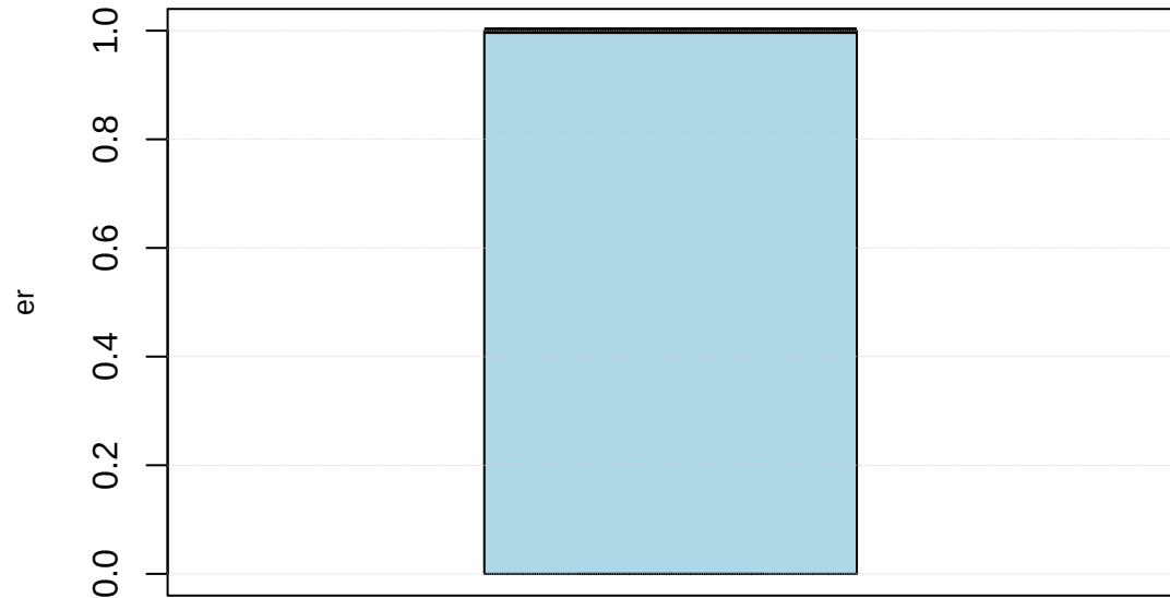
Boxplot of er
