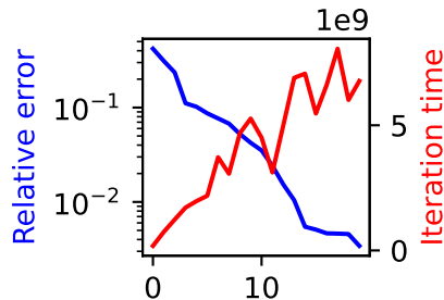
L=8 chi=7
