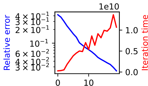
L=10 chi=5
