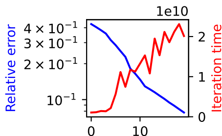
L=30 chi=7
