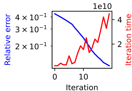
L=30 chi=9
