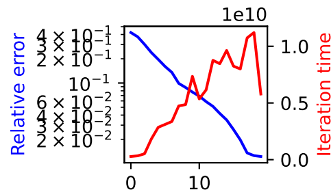
L=10 chi=9
