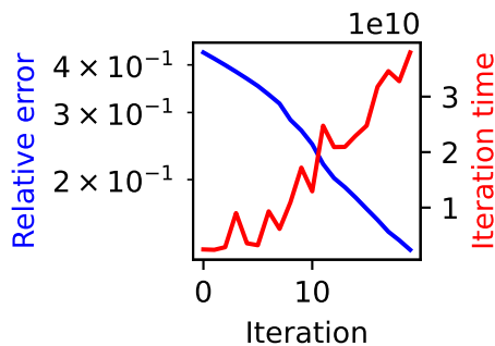
L=30 chi=7
