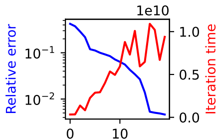
L=10 chi=7
