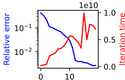
L=8 chi=5
