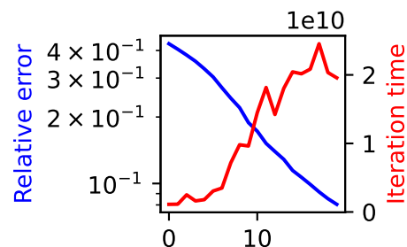
L=30 chi=9
