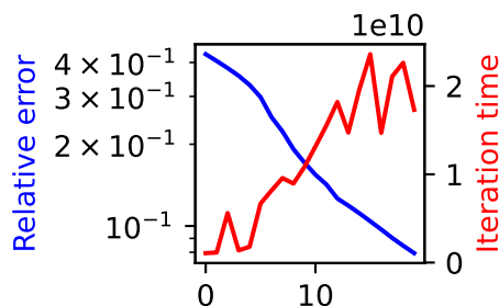
L=30 chi=5
