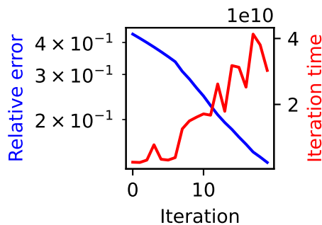
L=30 chi=5
