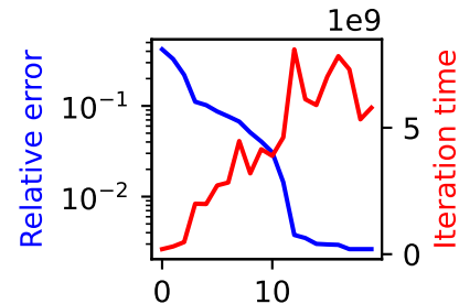
L=8 chi=9
