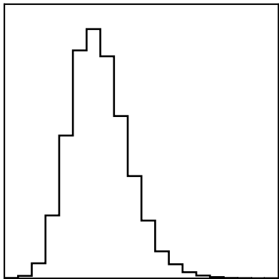
Dust Mass ( M_{\odot} )
