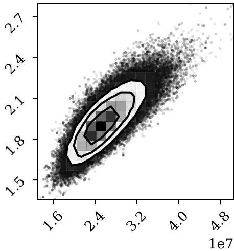
Dust Mass ( M_{\odot} )
