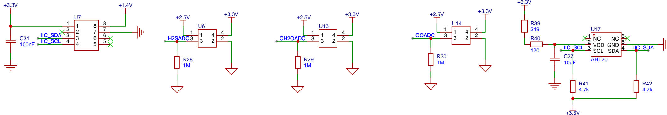
气体传感器电路
