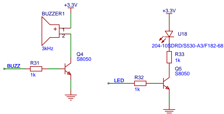
声光报警电路
