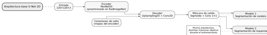
Figura 3.6: Esquema de la arquitectura U-Net 2D empleada en este trabajo. Fuente: elaboración propia.
