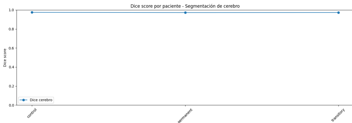
Figura 4.1: Evolución del coeficiente Dice por Caso en el estudio de segmentación del cerebro en modelo control y con ictus isquémico permanente y transitorio. Fuente: elaboración propia.
