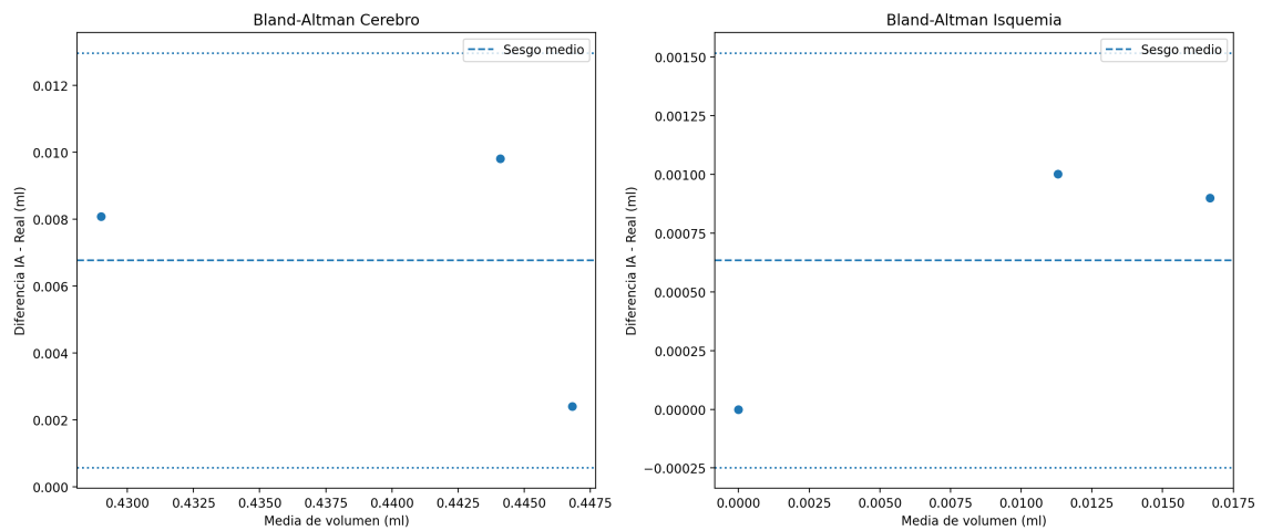
Figura 4.9: Gráfico de Bland-Altman para analizar la concordancia entre el volumen calculado manualmente y el volumen estimado por el modelo. Fuente: elaboración propia.
