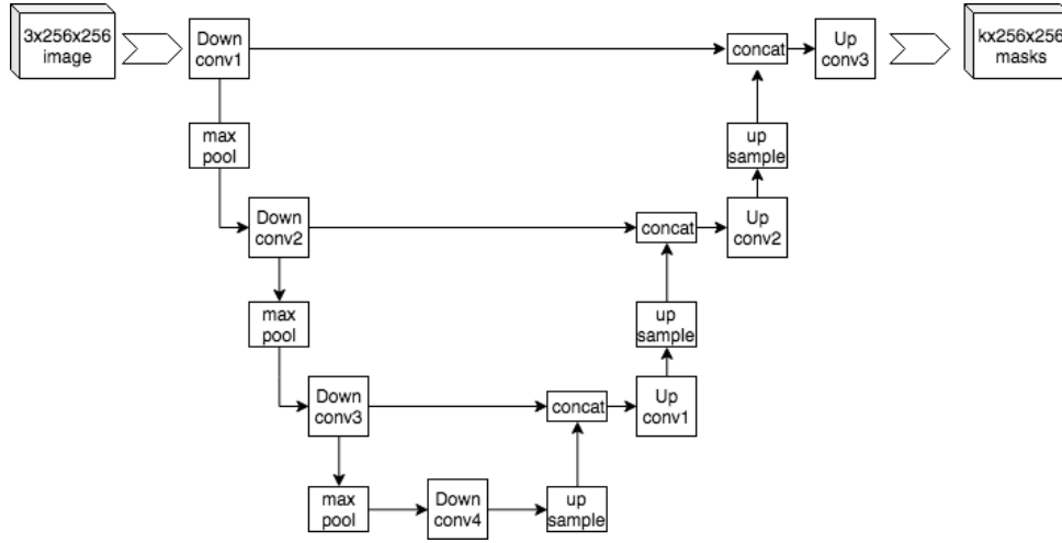
Figura 2.2: Ejemplo de arquitectura U-Net para segmentación de imágenes. Fuente: Mehrdad Yazdani, Wikimedia Commons, licencia CC BY-SA 4.0.
